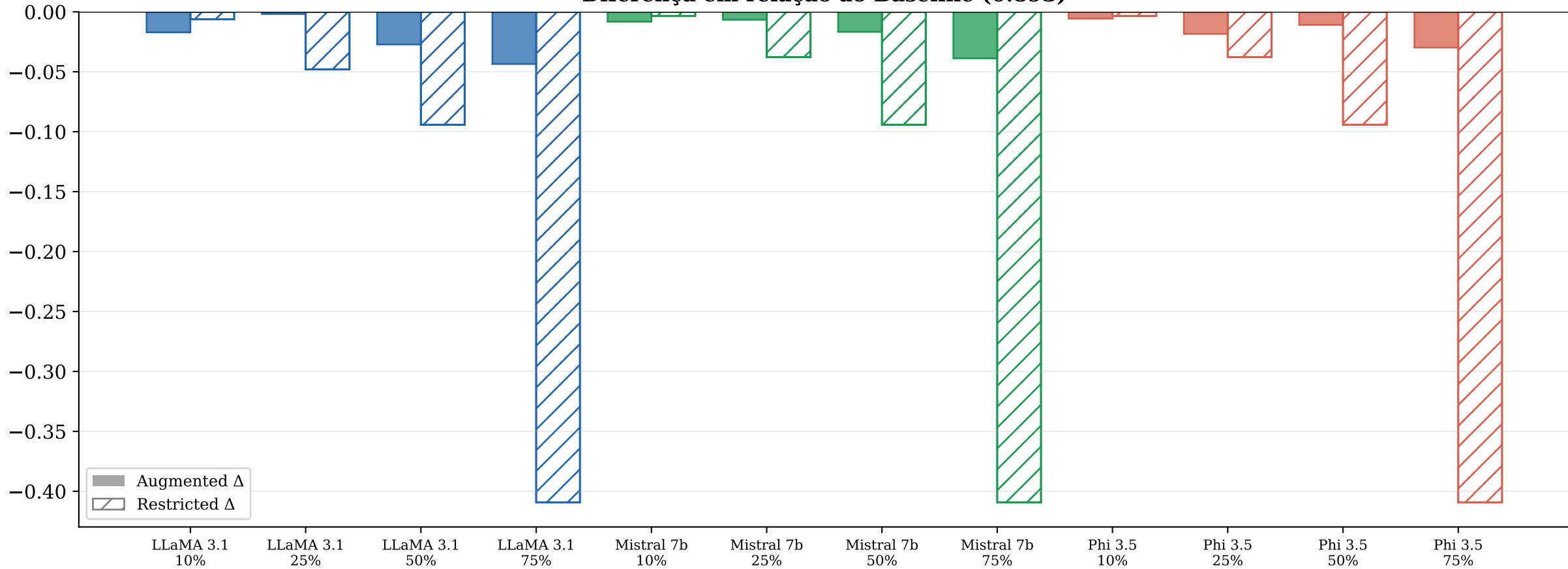
Diferença em relação ao Baseline (0.893)
