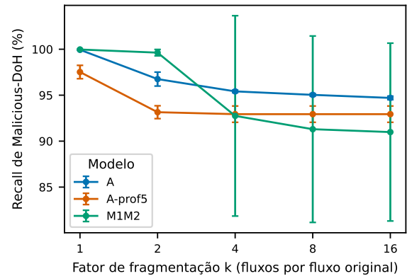
Fig. 5. Recall de Malicious-DoH sob fragmentação simulada do fluxo, no CIRA: duração e bytes dos fluxos maliciosos do teste divididos por k , sem retraining. A e A-prof5: sistema do artigo com profundidade variável e com profundidade 5; M1M2: modificação da equipe. 10 seeds, média \pm desvio padrão amostral.
