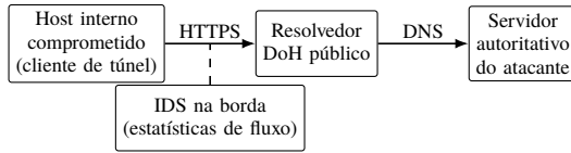
Fig. 1. Túnel DNS sobre DoH: os dados saem codificados em consultas DNS, dentro de HTTPS, até o servidor autoritativo que o atacante controla. O IDS observa o fluxo cifrado na borda da rede da organização.
