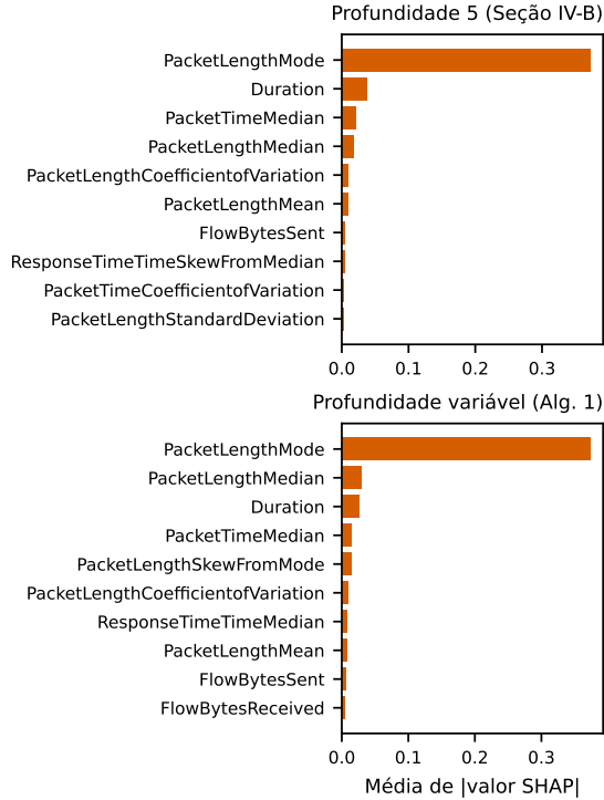
Fig. 4. Importância global dos 10 atributos de maior média do valor absoluto de SHAP para Malicious-DoH, equivalente à Fig. 5 do artigo, no Random Forest base 1, CIRA, nas duas leituras de profundidade. Amostra de 2000 fluxos por classe do treino; seed 42.
