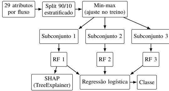
Fig. 2. Sistema do artigo. Cada subconjunto recebe um terço do Non-DoH, todo o Malicious-DoH e o Benign-DoH aumentado com SMOTE até igualar o Malicious-DoH.
