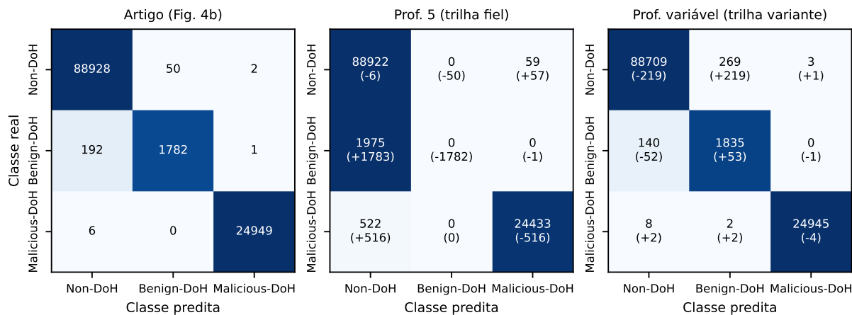
Fig. 3. Matrizes de confusão no teste: artigo (Fig. 4b) e reprodução nas duas leituras de profundidade. Em cada célula, o número de fluxos e, entre parênteses, a diferença para o artigo. Seed 42.
