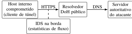
Fig. 1. Túnel DNS sobre DoH: os dados saem codificados em consultas DNS, dentro de HTTPS, até o servidor autoritativo que o atacante controla. O IDS observa o fluxo cifrado na borda da rede da organização.
