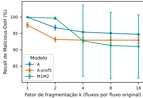
Fig. 5. Recall de Malicious-DoH sob fragmentação simulada do fluxo, no CIRA: duração e bytes dos fluxos maliciosos do teste divididos por k , sem retreino. 10 seeds, média \pm desvio padrão amostral.
