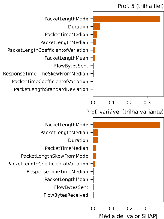
Fig. 4. Importância global dos 10 atributos de maior média do valor absoluto de SHAP para Malicious-DoH, equivalente à Fig. 5 do artigo, no Random Forest base 1, CIRA. Amostra de 2000 fluxos por classe do treino; seed 42.
