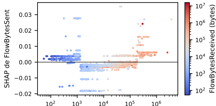
(b) FlowBytesSent (bytes, escala logarítmica)
