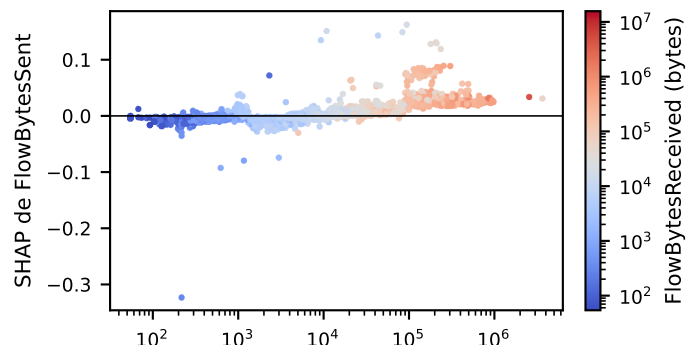
(b) FlowBytesSent (bytes, escala logarítmica)
