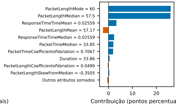
Fig. 8, prof. variável: Non-DoH média 37.3% → predição 100.0%
