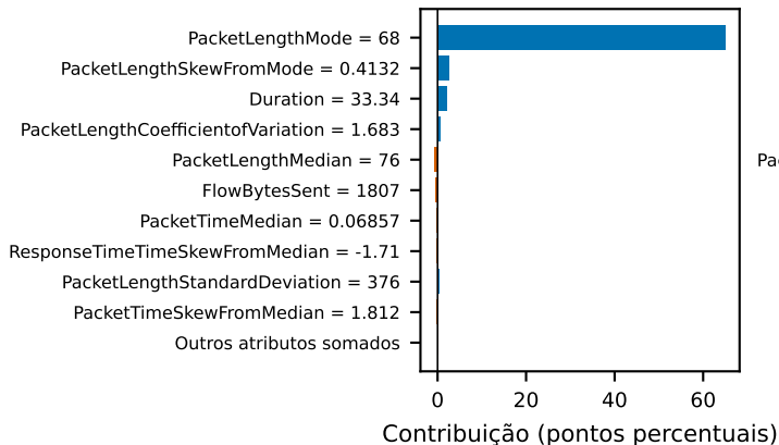
Fig. 7, prof. variável: Malicious-DoH média 31.4% → predição 100.0%
