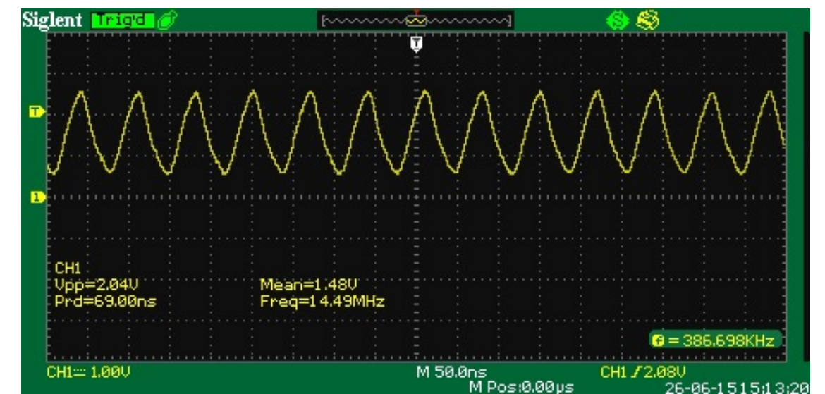
IC16 Pin 6 TCLK input
