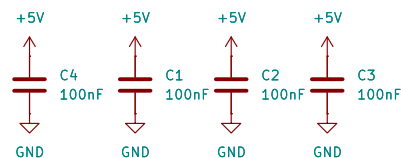
Decoupling
