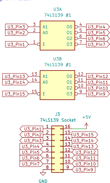
Original 74LS139
