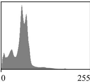
a) Original
