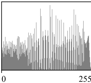
c) Global
