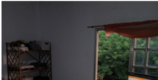
a) Original
