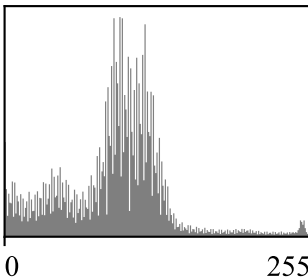
b) Estiramiento
