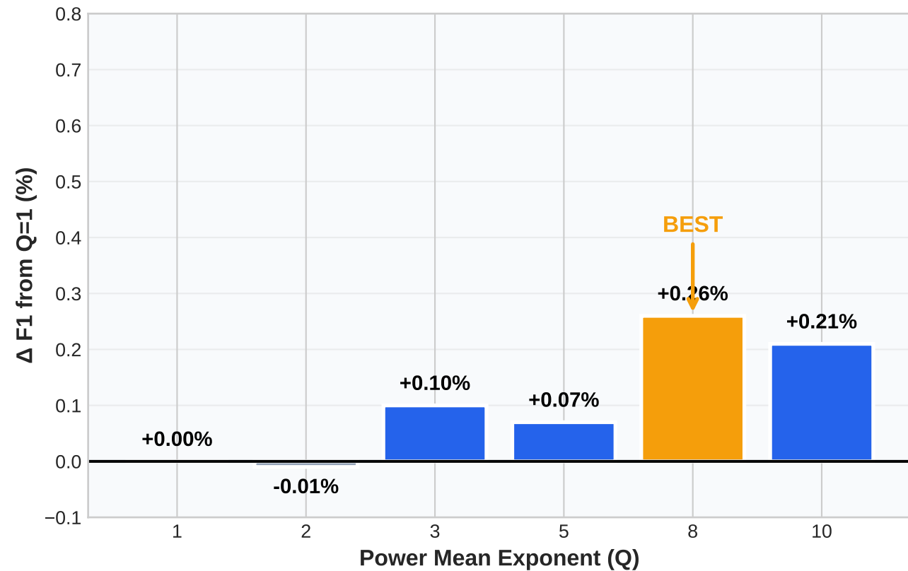
(b) F1 Improvement vs Arithmetic Mean (Q=1)
