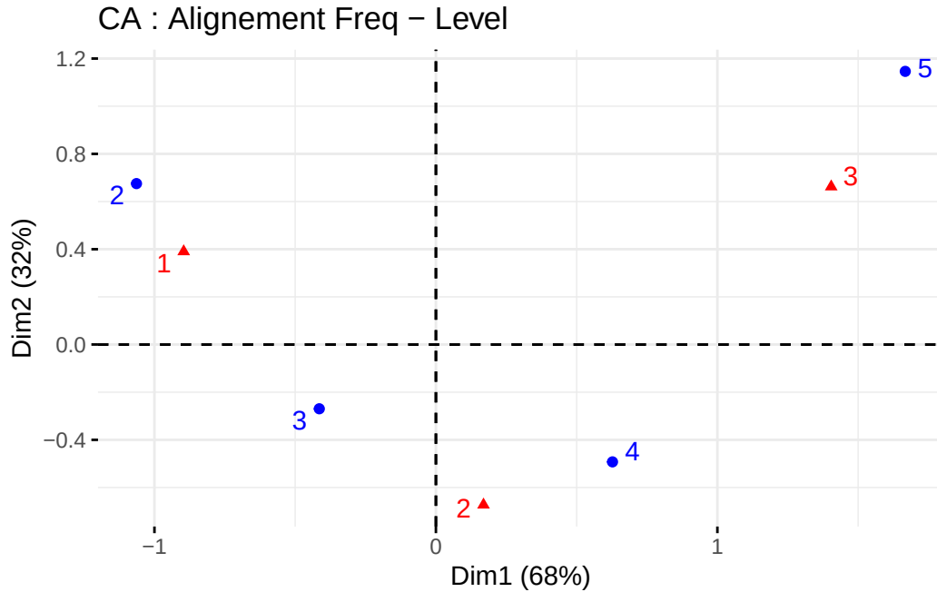
Figure 1: Projection des différentes modalités Level et Freq sur le premier plan factorielle
