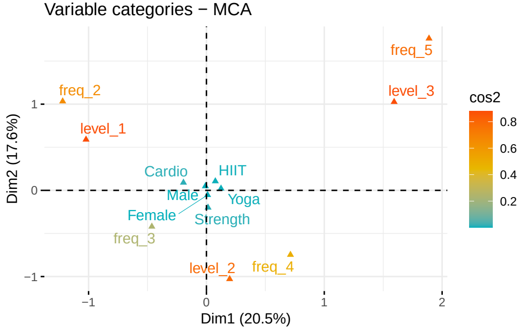
Figure 2: Projection des différentes modalités sur le premier plan factorielle
