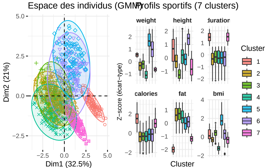
FIGURE 5 : Profils des 7 classes (Mélanges) . Distribution des variables standardisées par cluster.
