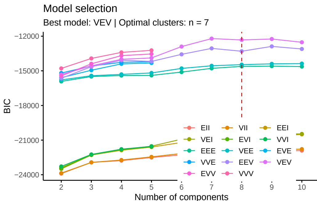
FIGURE 4 : Sélection du modèle (BIC/ICL). Le modèle VEV à 7 composantes minimise la perte d'information.
