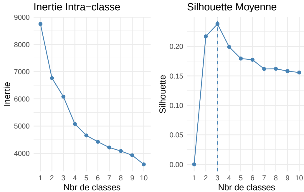
FIGURE 1 : Méthode du coude et Silhouette
