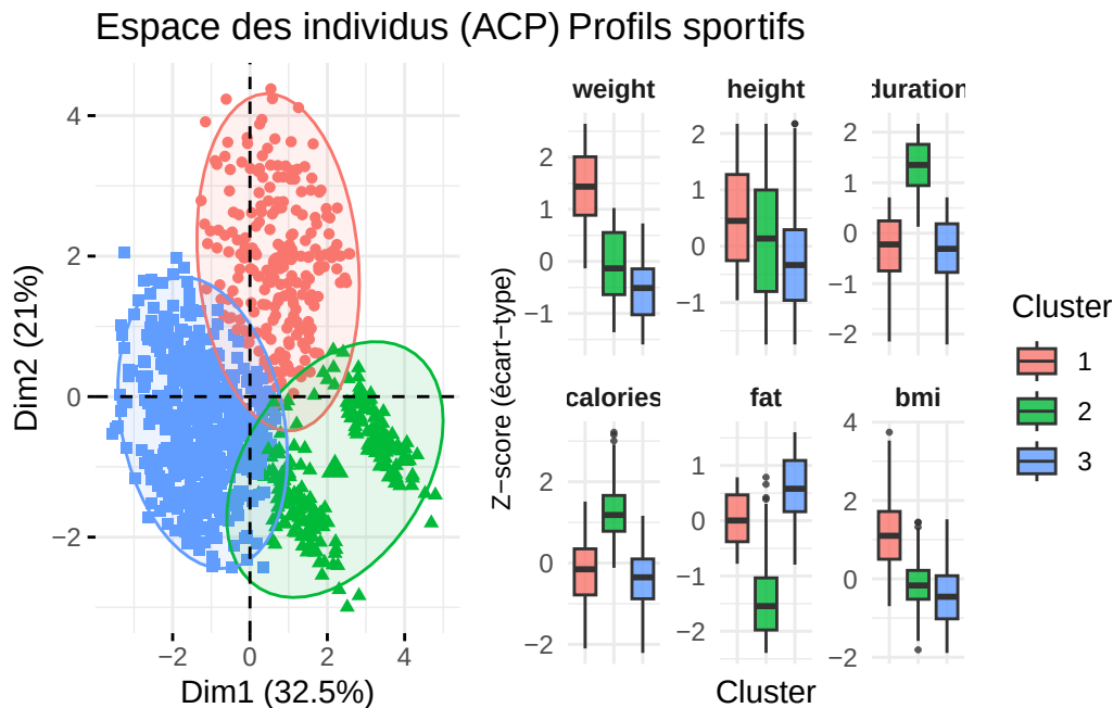
FIGURE 3 : Caractérisation des clusters retenus (K=3) . Gauche : Projection sur le plan factoriel. Droite : Boxplots des variables discriminantes.
