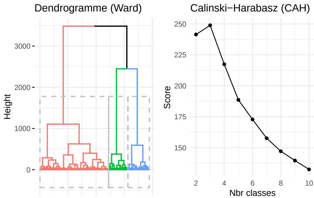
FIGURE 2 : Critères de sélection du nombre de classes. Gauche : Dendrogramme de la CAH. Droite : Méthode de Calinski-Harabasz.
