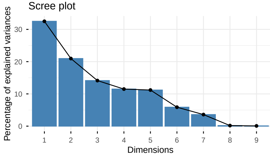
FIGURE 5 – Pourcentage de variance expliquée par dimension
