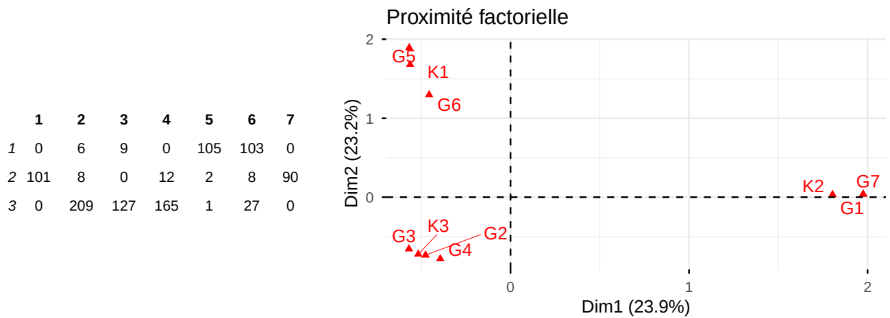
FIGURE 17 – Analyse croisée des partitions. Gauche : Matrice de confusion. Droite : Plan factoriel MCA.
