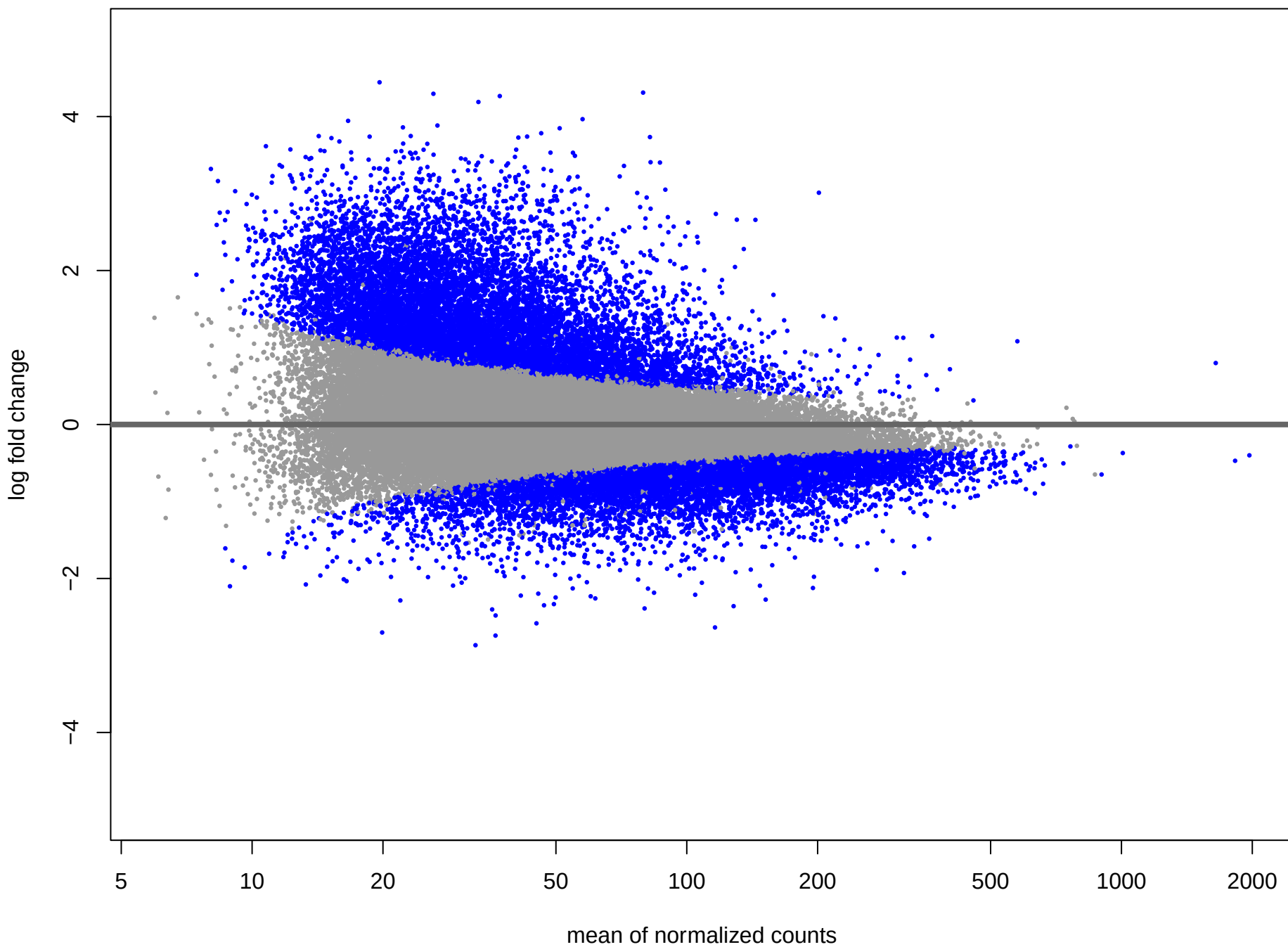
MA Plot: HFD vs CHD
