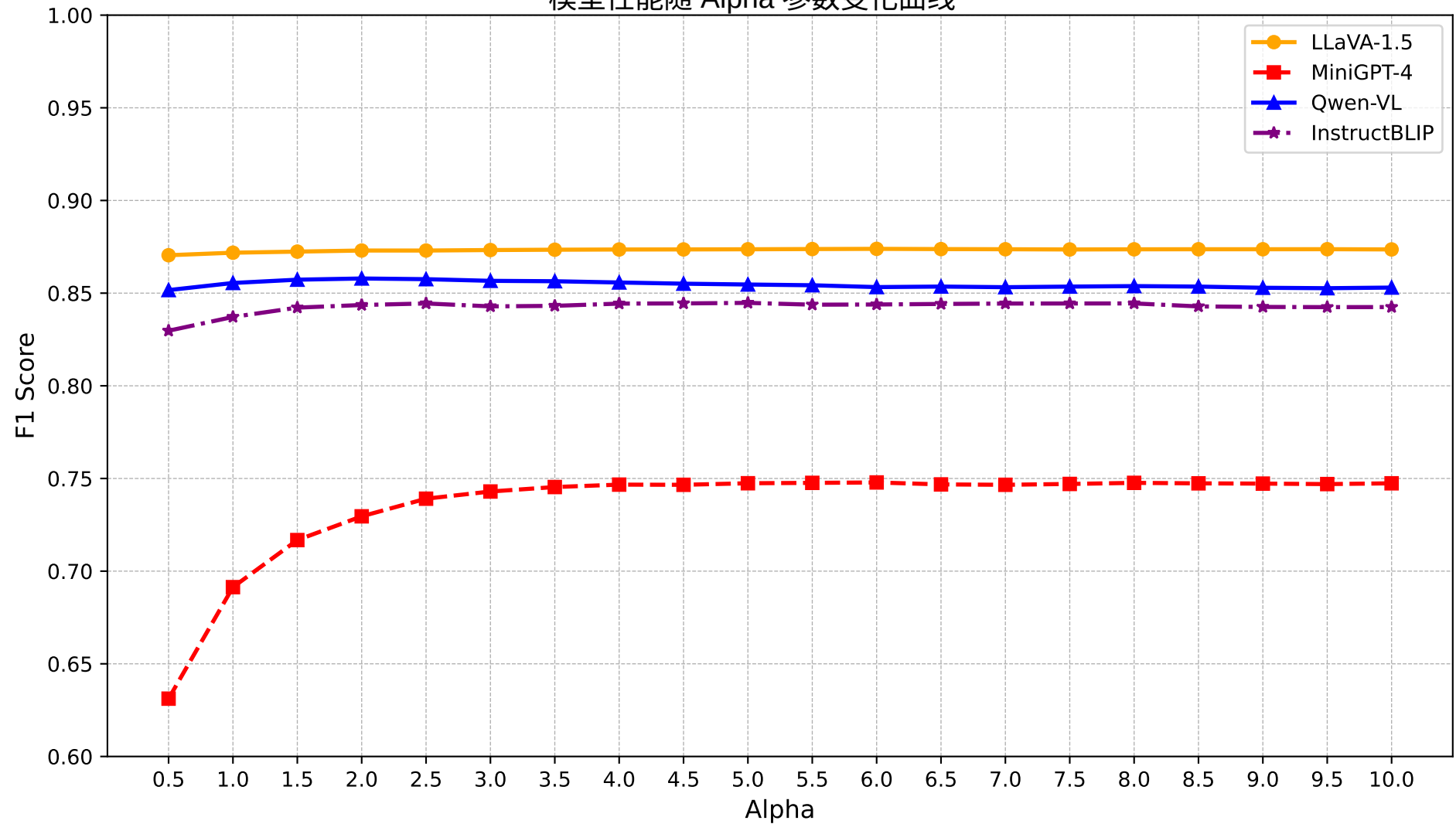
模型性能随 Alpha 参数变化曲线
