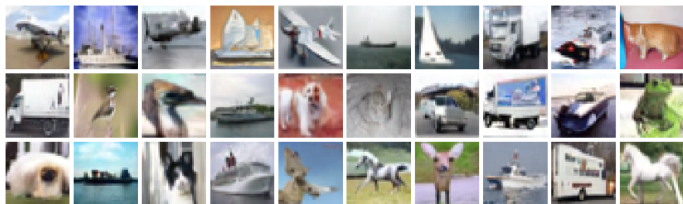
NF (rKL)
