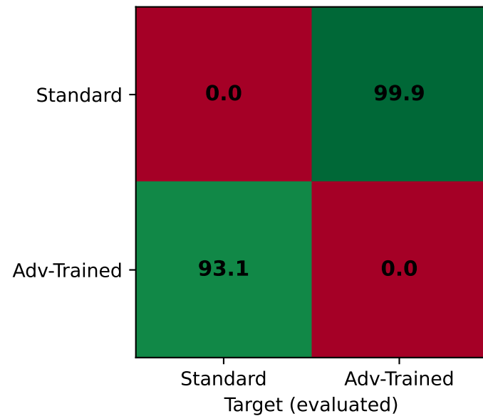
C&W
