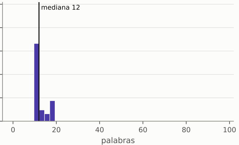
VL-JEPA · p4m
