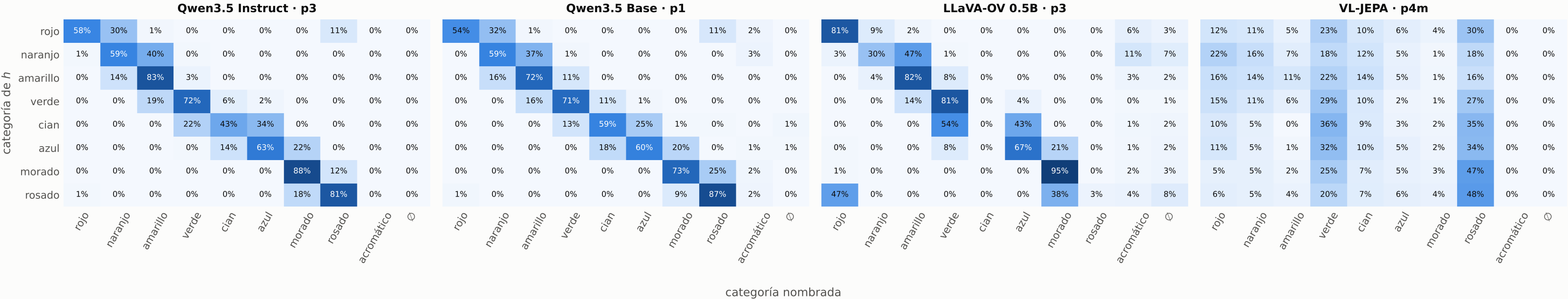
Figura 9 — Confusión de categoría de color (normalizada por fila)
