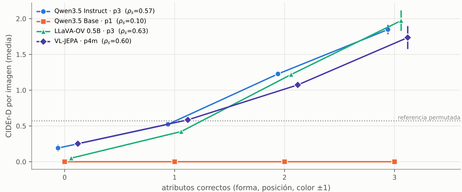
Figura 12 — CIDEr-D (texto normalizado) según la fidelidad
