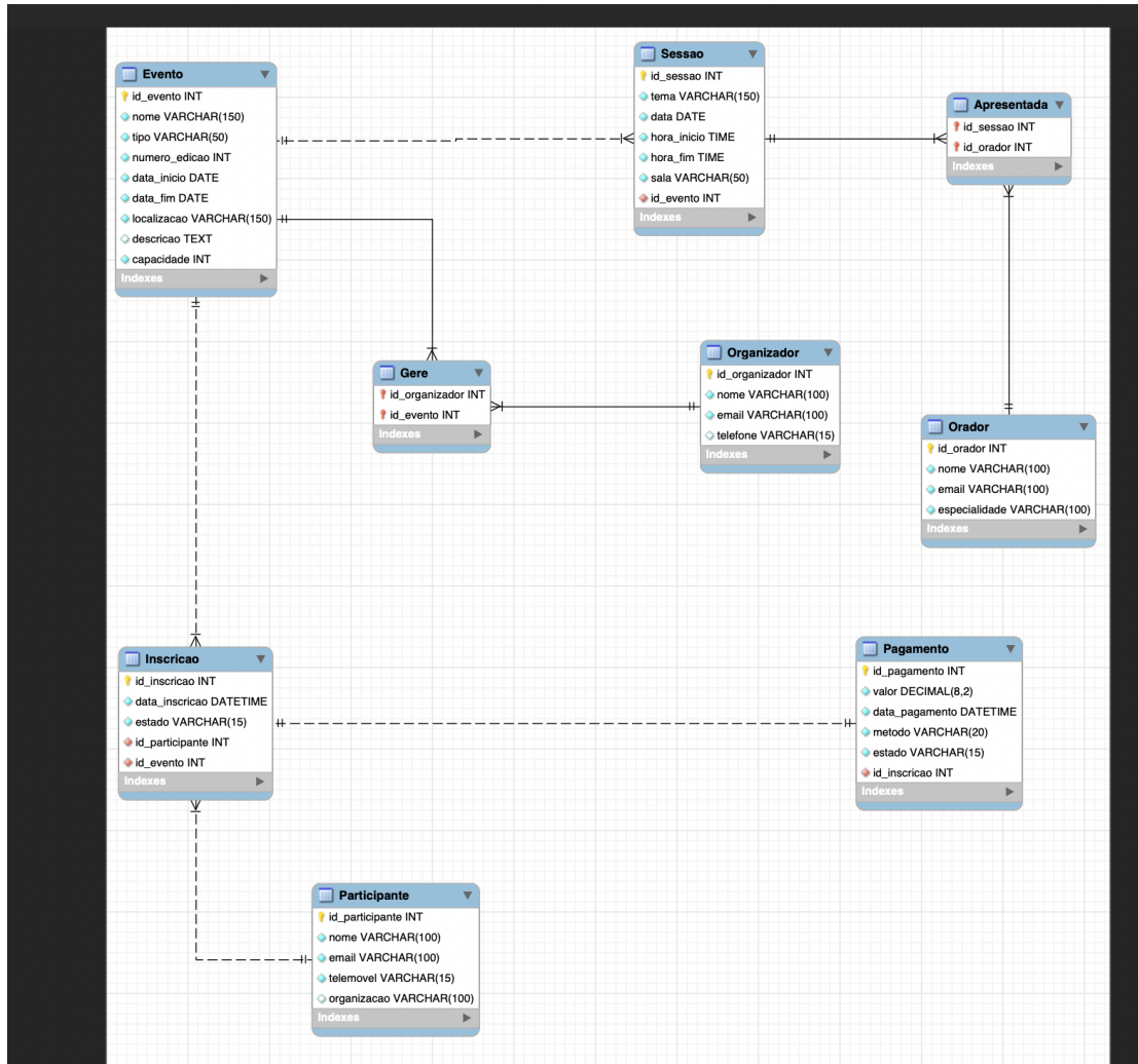
Figura 11. Modelo lógico do sistema EvenSync (gerado com MySQL Workbench)
