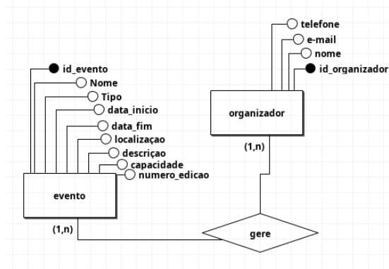
Figura 5. Relacionamento gere entre Organizador e Evento
