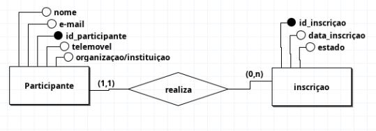
Figura 2. Relacionamento realiza entre Participante e Inscrição
