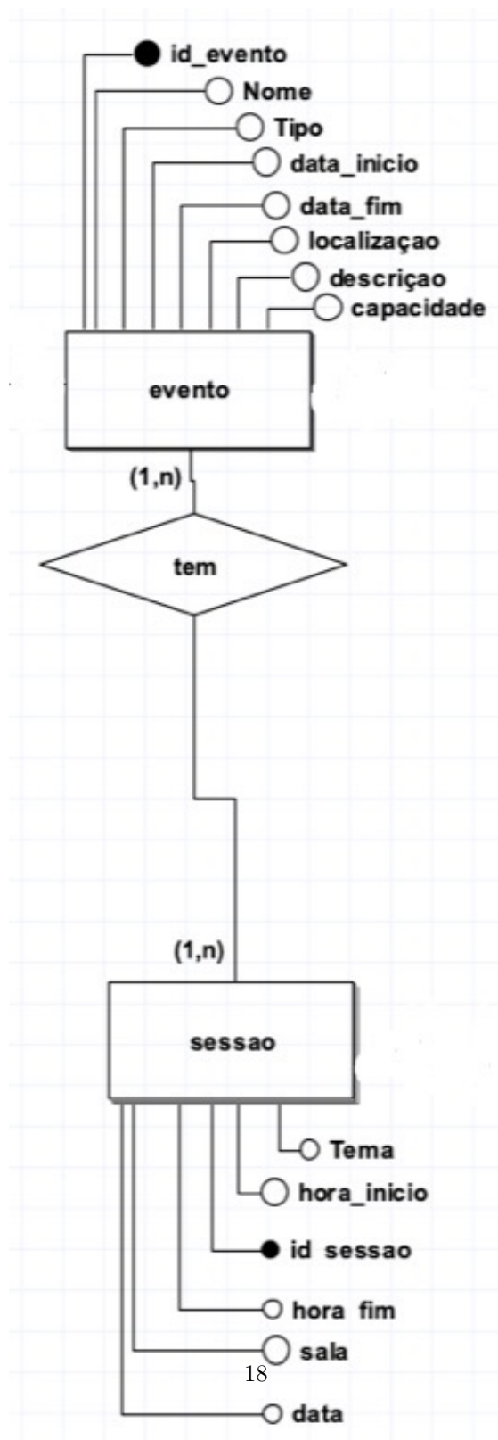
Figura 5. Relacionamento tem entre Evento e Sessão
