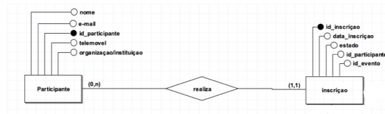
Figura 1. Relacionamento realiza entre Participante e Inscrição
