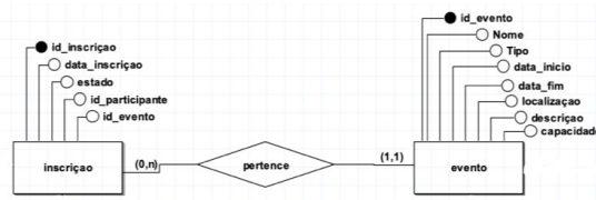
Figura 2. Relacionamento pertence entre Inscrição e Evento
