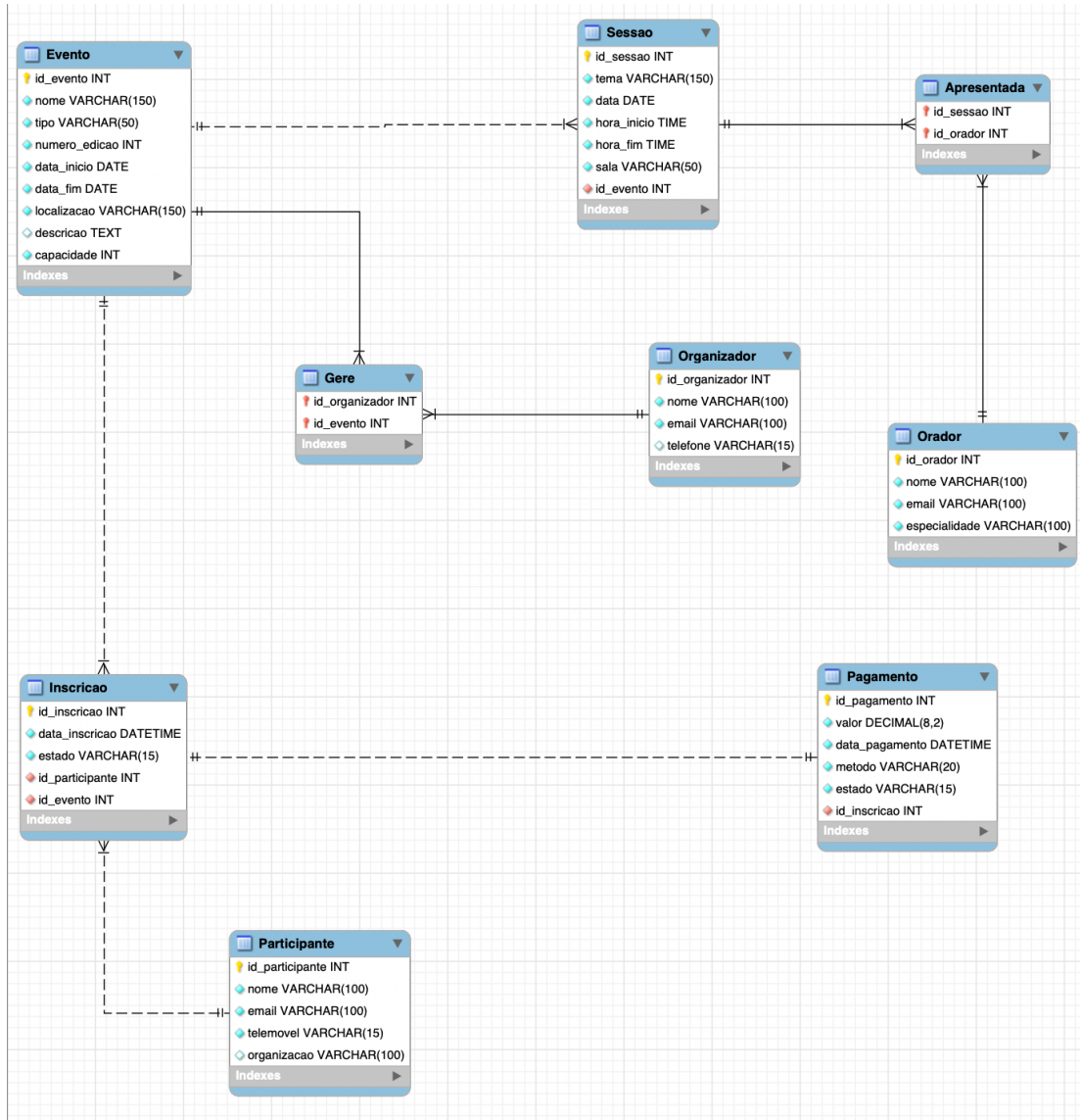
Figura 11. Modelo lógico do sistema EvenSync (gerado com MySQL Workbench)
