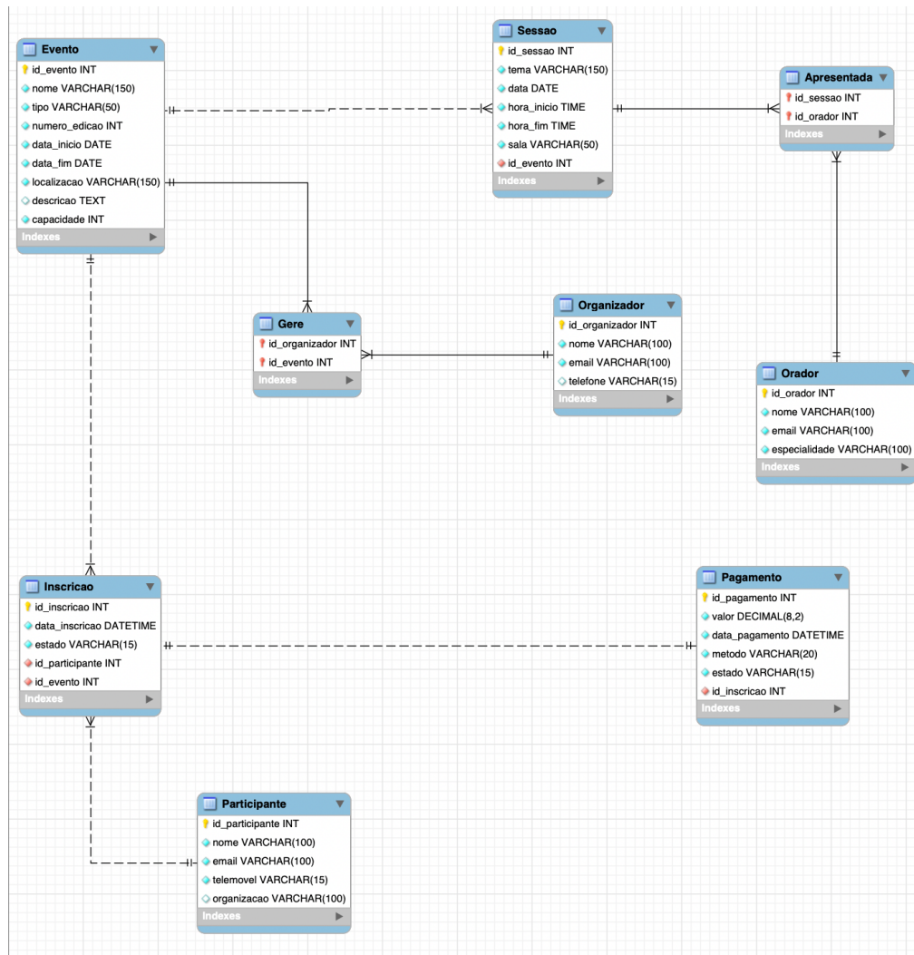
Figura 9. Diagrama do Modelo Lógico do sistema EvenSync (gerado com MySQL Workbench)
