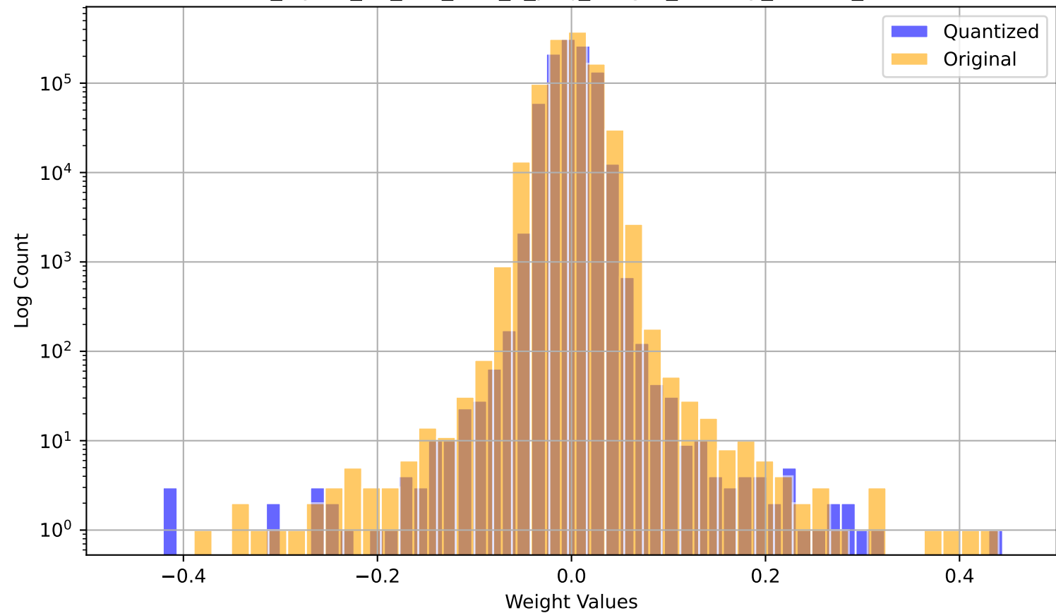
model_layers_31_self_attn_o_proj_weight_overlay_2.2652_2.0635
