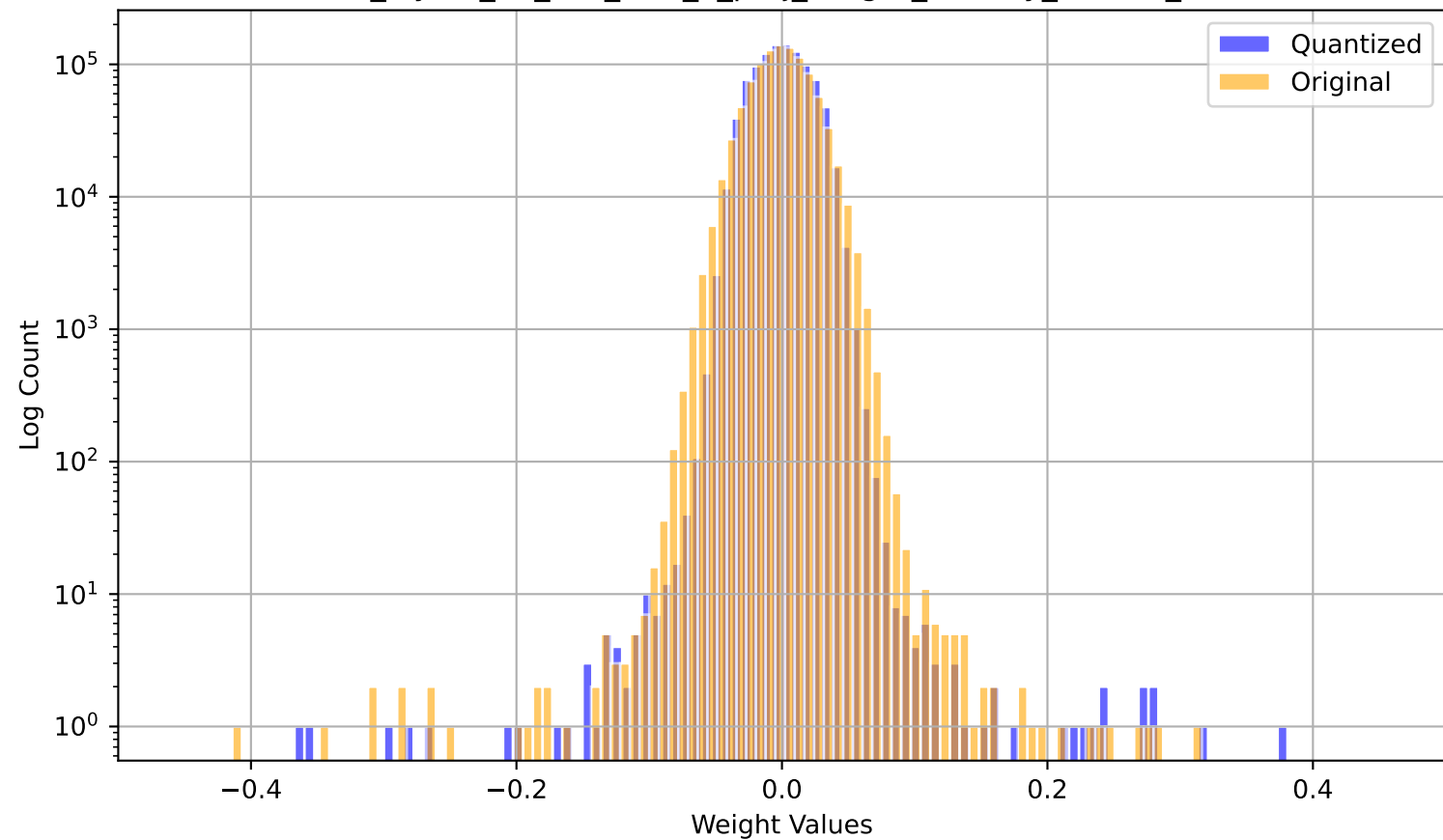
model_layers_30_self_attn_o_proj_weight_overlay_2.9517_2.9674
