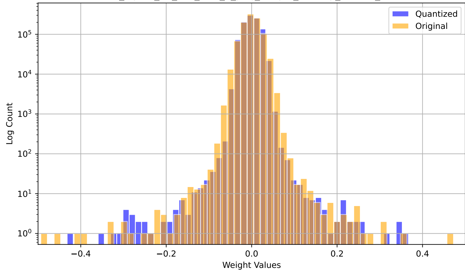
model_layers_31_self_attn_o_proj_weight_overlay_2.1571_2.0635
