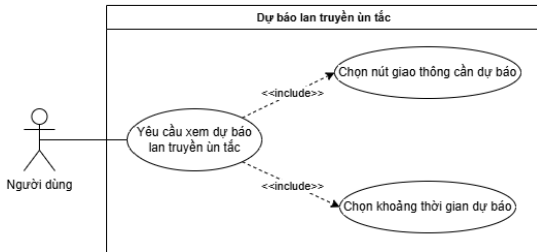
Hình 20: Sơ đồ Use Case dự báo ứn tắc giao thông
