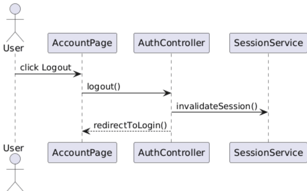
Hình 27: Sơ đồ Sequence đăng xuất
