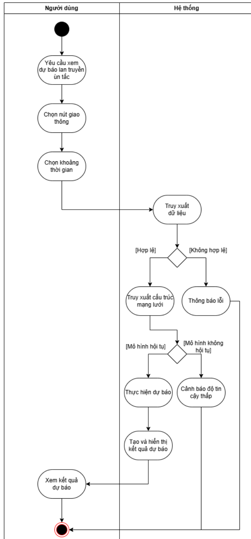
Hình 25: Sơ đồ Activity dự báo lan truyền ùn tắc giao thông
