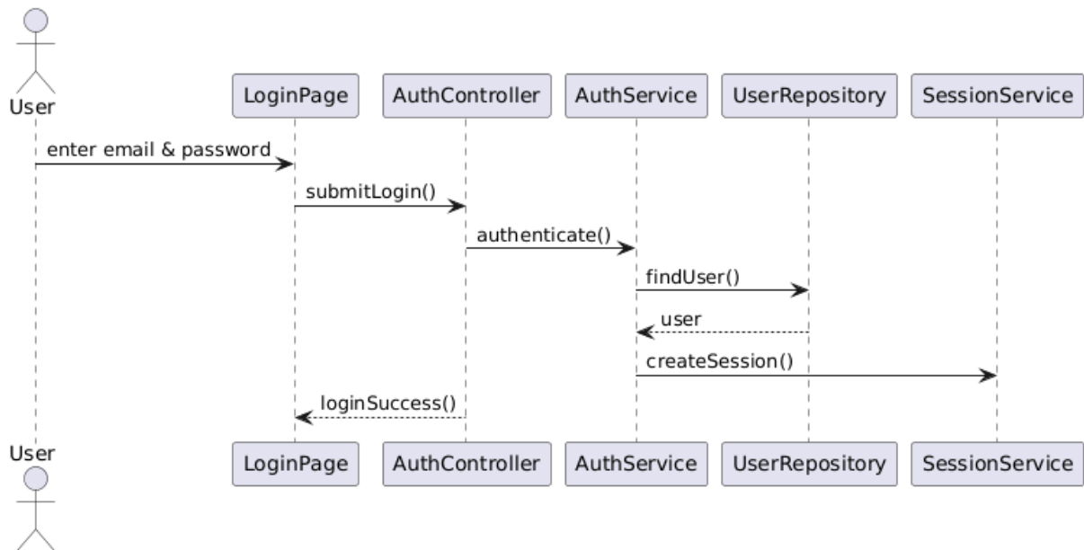
Hình 26: Sơ đồ Sequence đăng nhập
