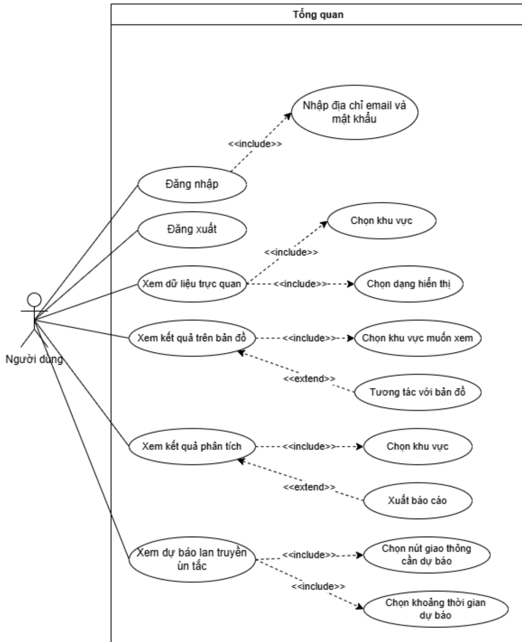
Hình 15: Sơ đồ Use Case tổng quan
