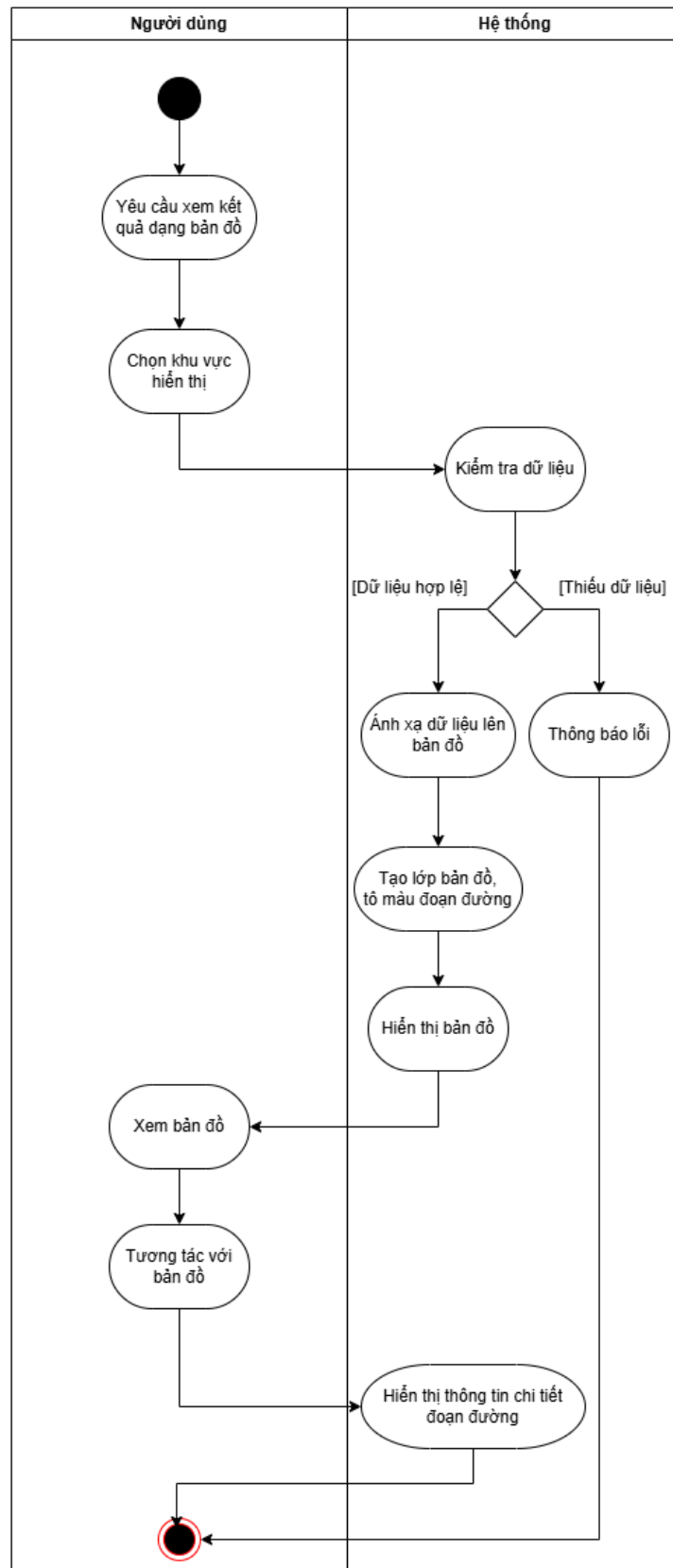
Hình 23: Sơ đồ Activity xem kết quả dạng bản đồ
