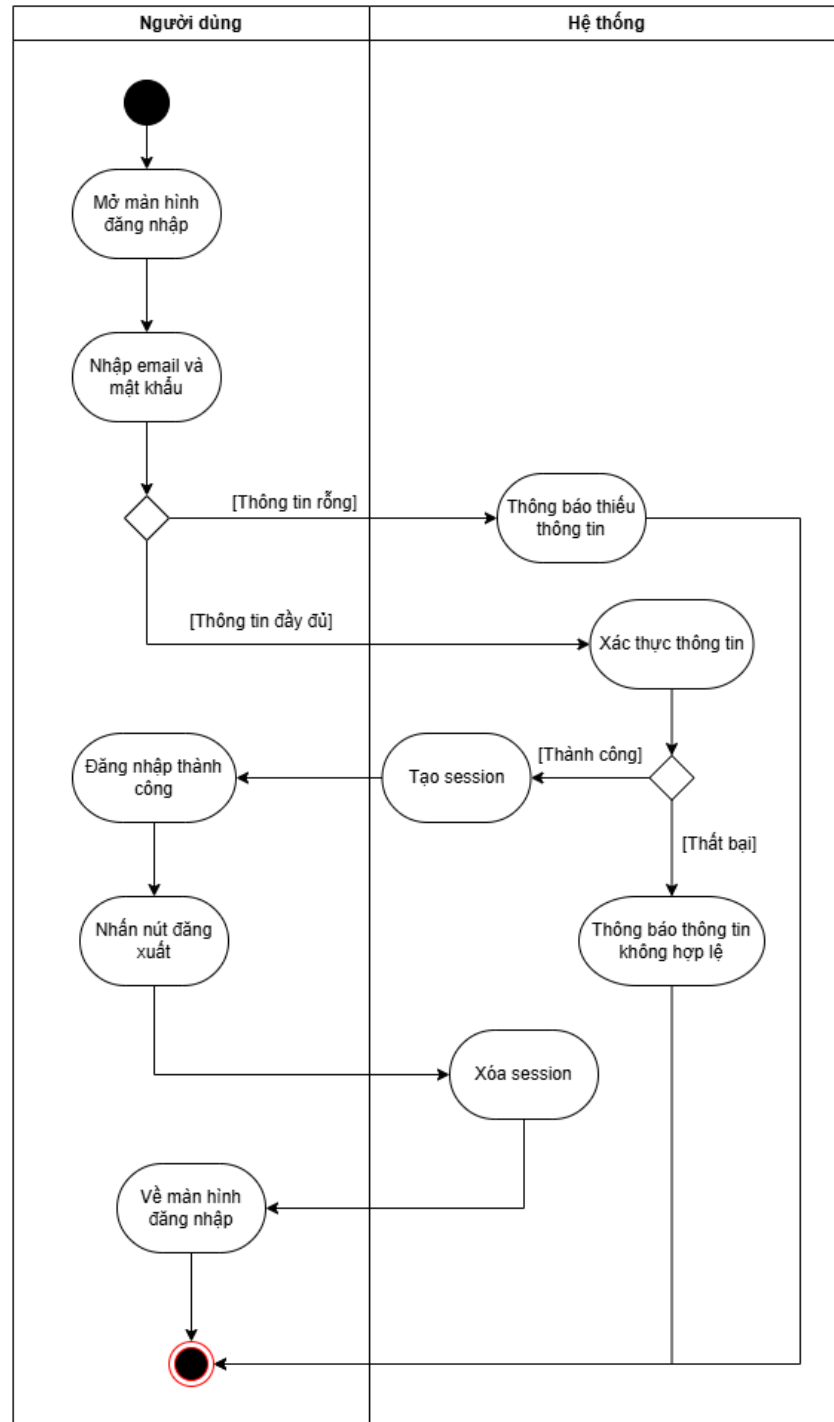
Hình 21: Sơ đồ Activity đăng nhập, đăng xuất
