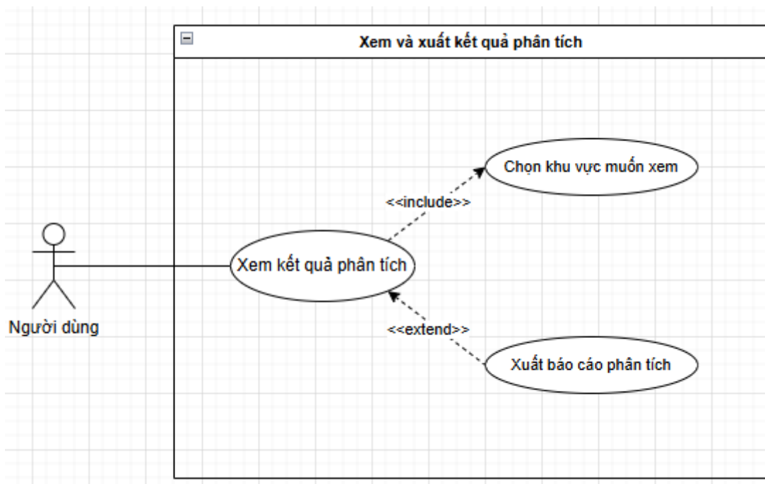
Hình 19: Sơ đồ Use Case xem và xuất kết quả phân tích
