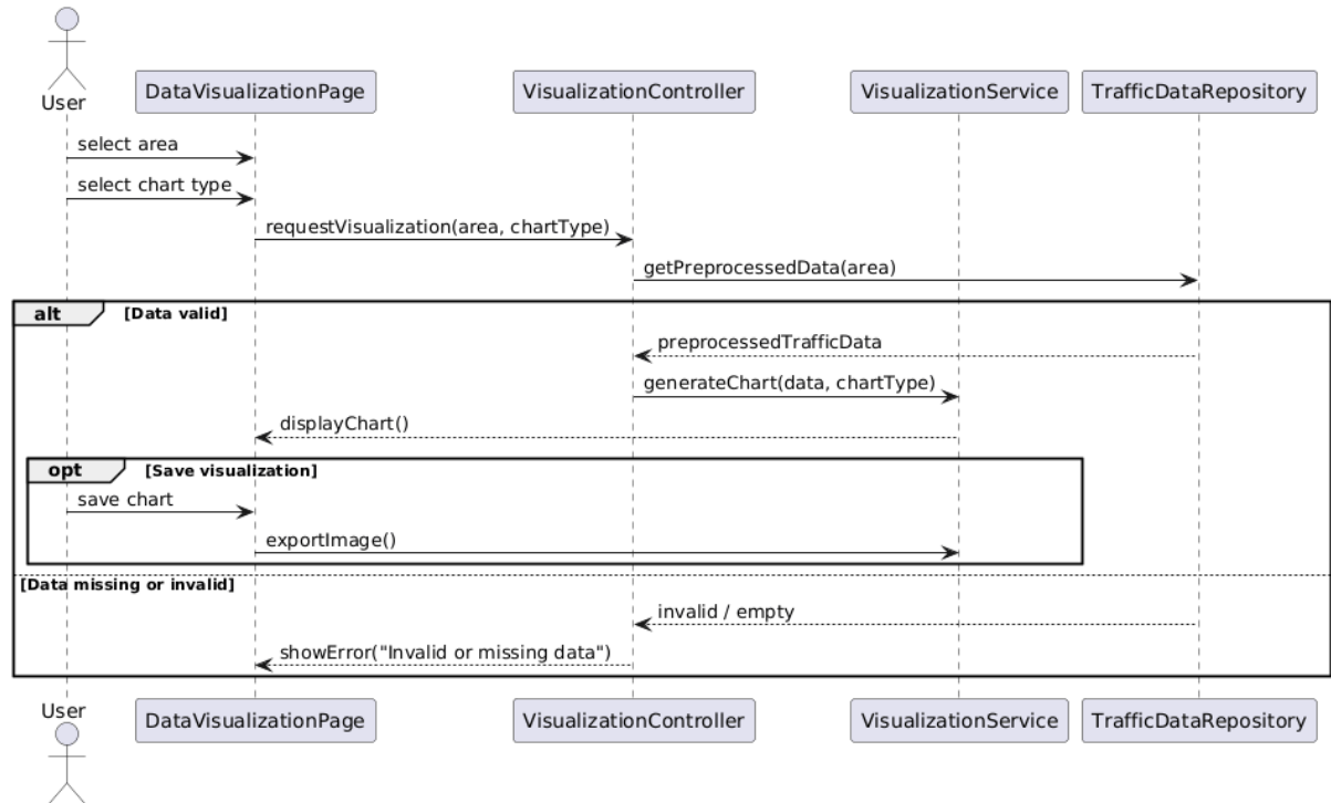
Hình 28: Sơ đồ Sequence trực quan hóa dữ liệu
