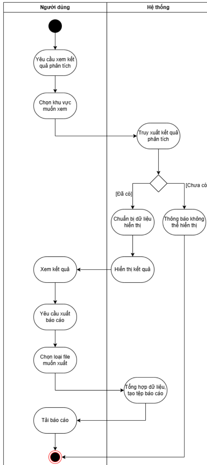
Hình 24: Sơ đồ Activity xem và xuất kết quả phân tích
