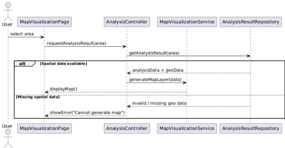
Hình 29: Sơ đồ Sequence xem kết quả dạng bản đồ
