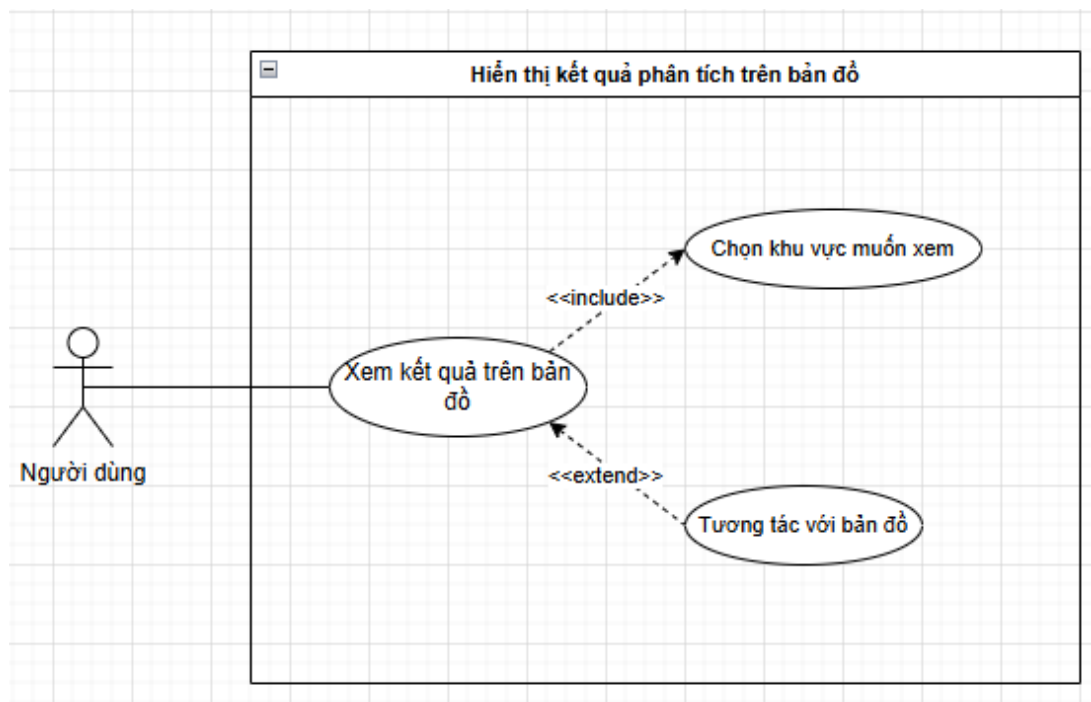
Hình 18: Sơ đồ Use Case hiển thị kết quả phân tích trên bản đồ
