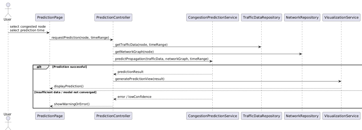
Hình 32: Sơ đồ Sequence dự báo lan truyền ùn tắc giao thông
