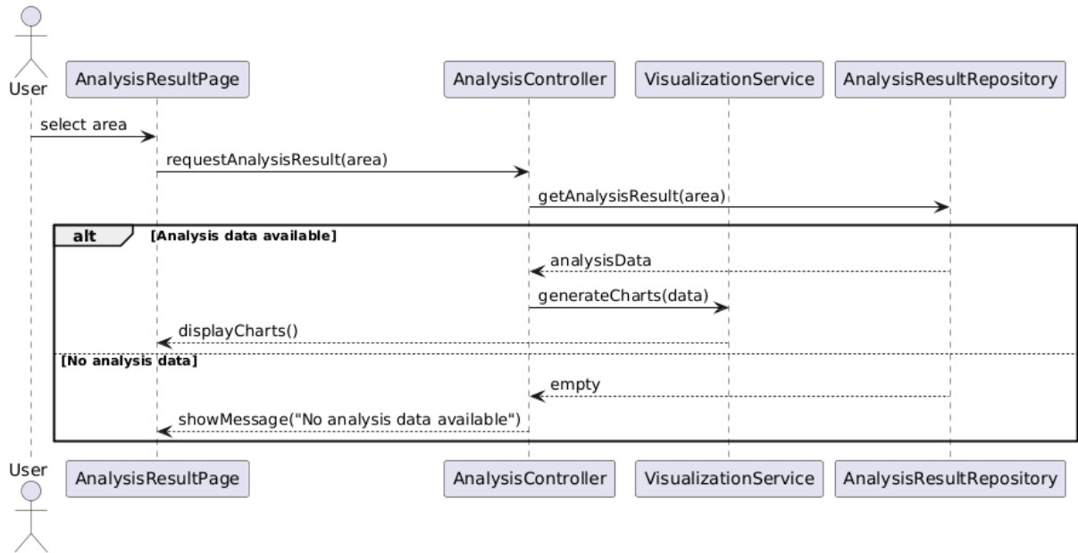
Hình 30: Sơ đồ Sequence xem kết quả phân tích
