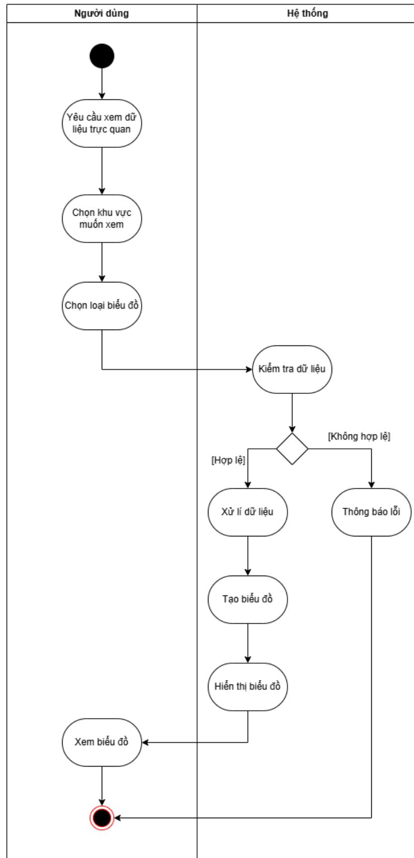
Hình 22: Sơ đồ Activity trực quan hóa dữ liệu
