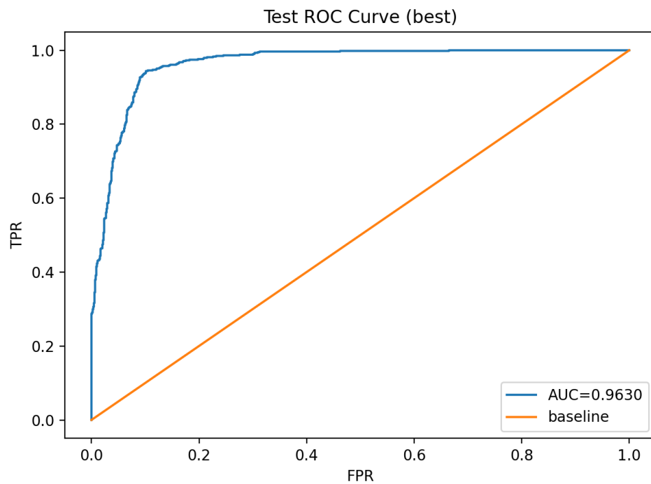
Hình 9: ROC, AUC
