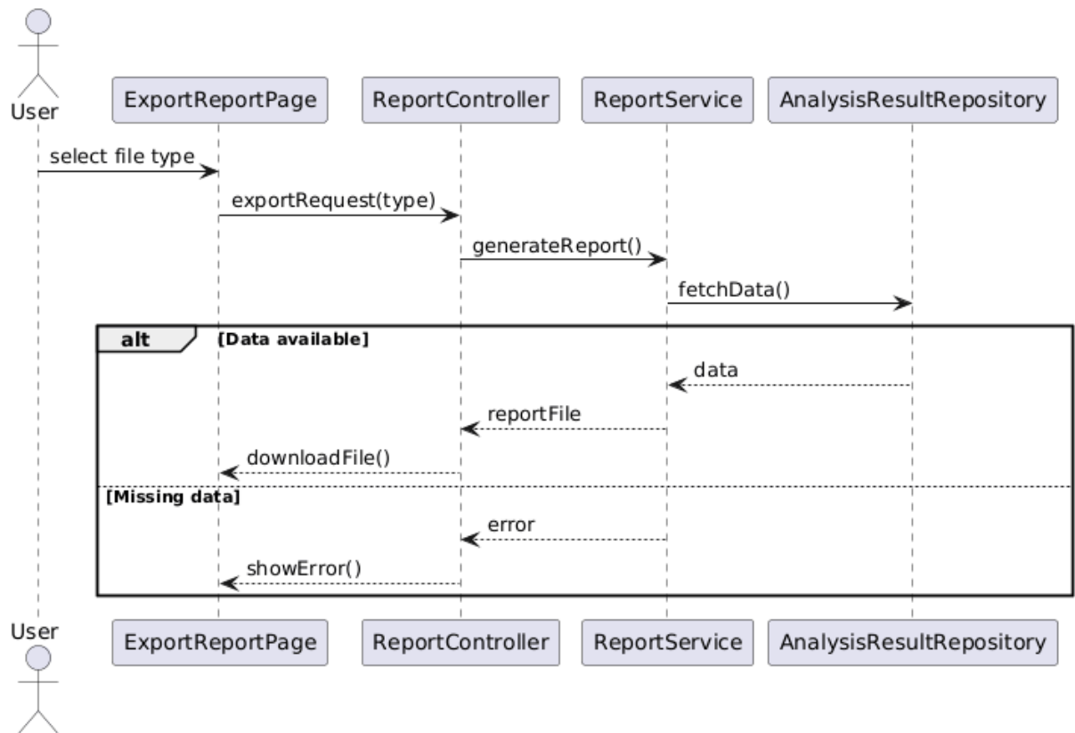
Hình 31: Sơ đồ Sequence xuất kết quả phân tích
