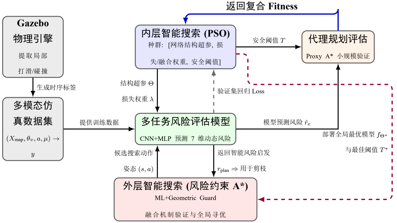
图 2: 机器学习与搜索双向嵌套协同架构
