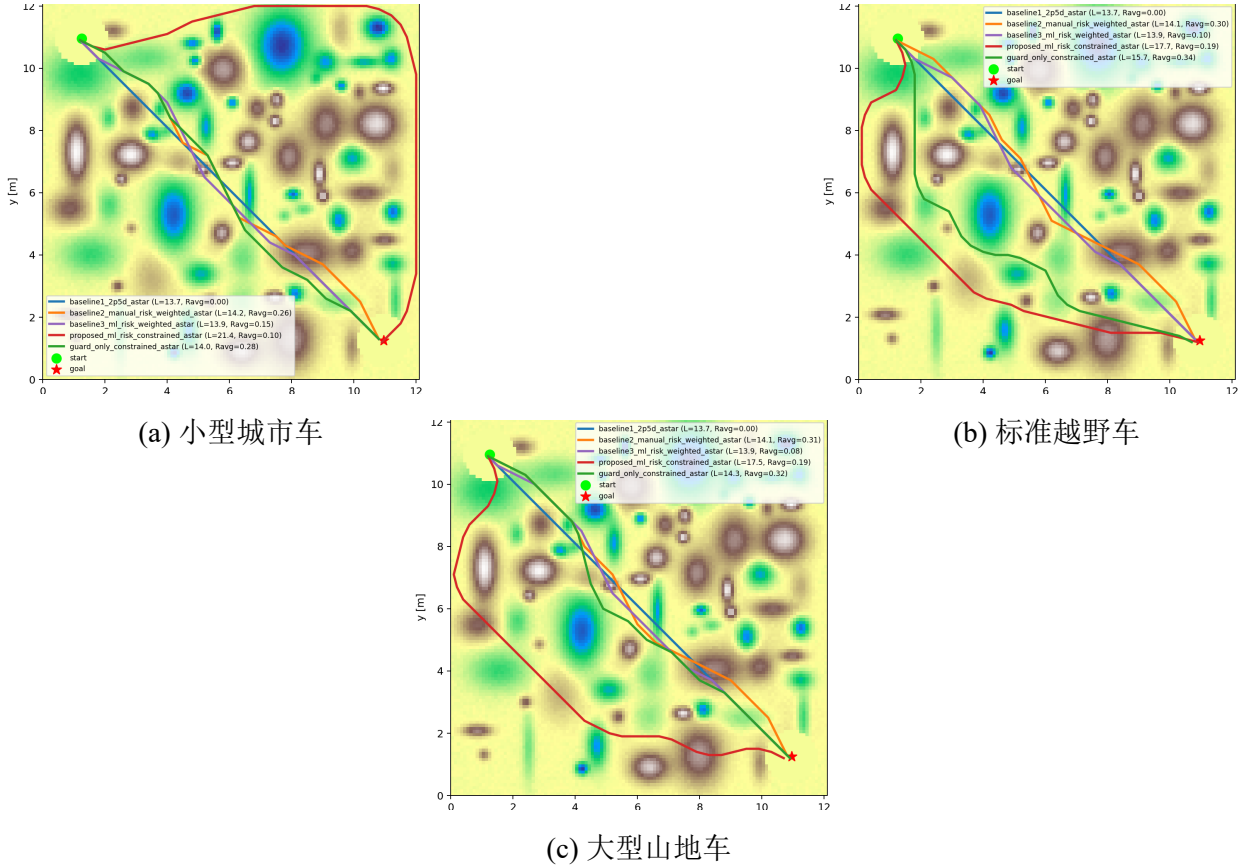
图 4: 同一散落障碍地形下不同车型的规划路径对比，红线为本方案
