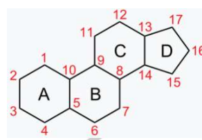
图 2 甾体化合物母核编号
