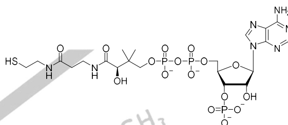
辅酶A的结构
