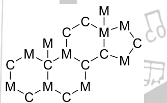
图 1 胆固酵母核中碳原子来源
