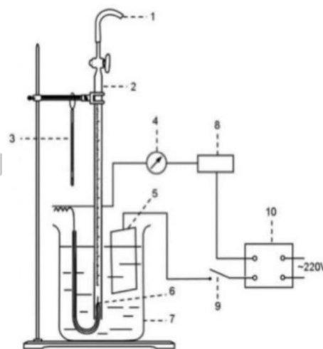
实验装置图
