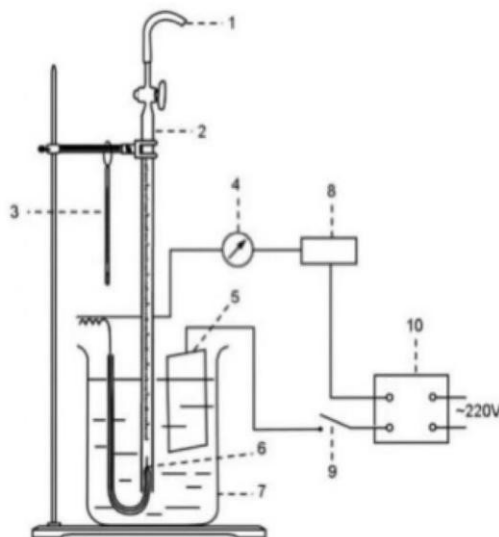
实验装置图
