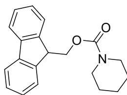
Fmoc-哌啶
