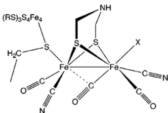
图 6.1 [\text{FeFe}] -氢化酶的活性位点的结构
