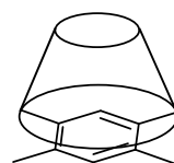
轴向结合
