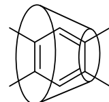
赤道结合
