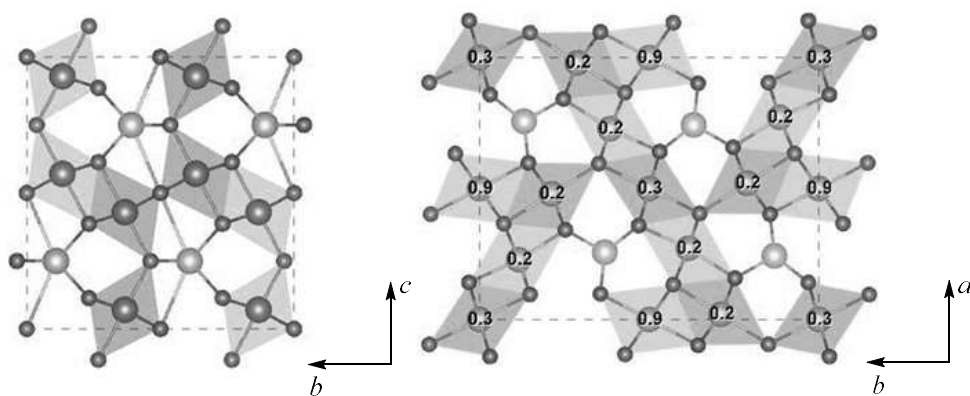
高压下 \text{MgCr}_2\text{O}_4
