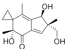
Illudin
