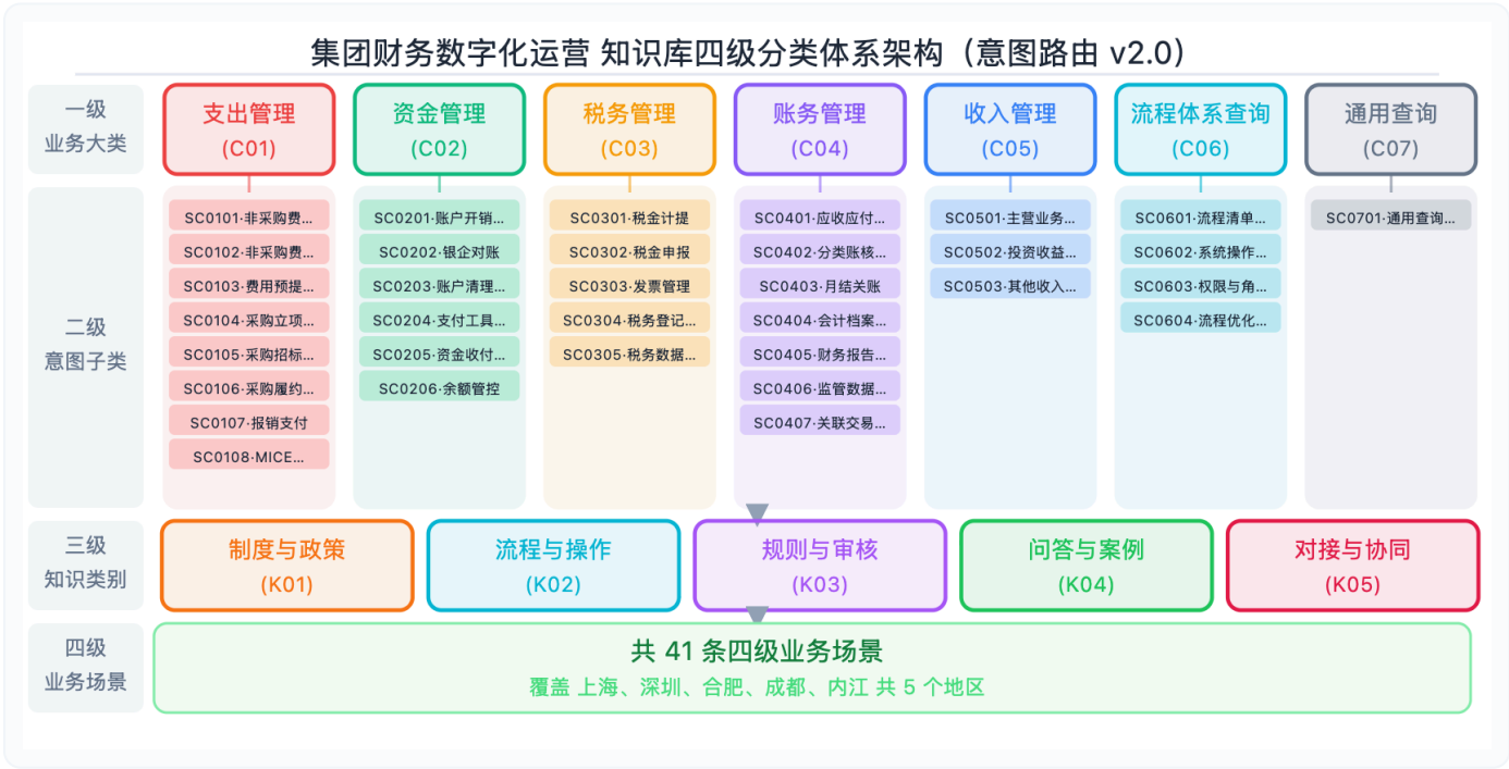
图1-0 集团财务数字化运营 知识库四级分类体系架构（意图路由 v2.0）
