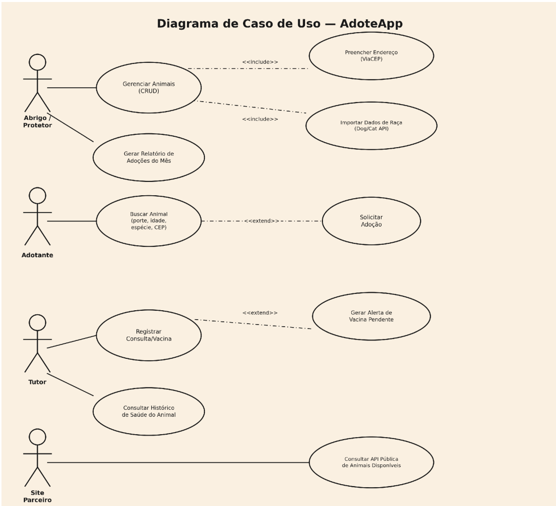
Figura 1 — Diagrama de casos de uso (UML) do AdoteApp.
