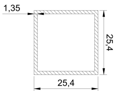
Tubo 1x1
