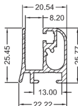
SP – 0293 Leito de 8mm
