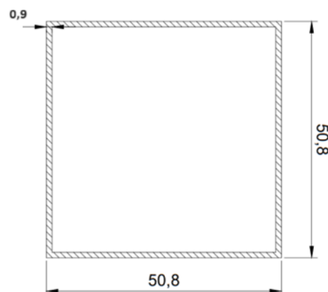
Tubo 2x2 SUPER LEVE
