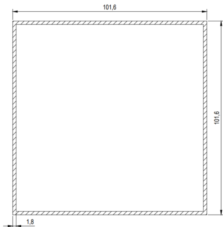
Tubo 4x4
