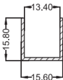
Perfil U – 5/8
