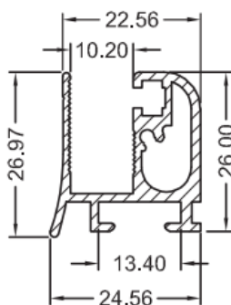
SP – 0294 Leito de 10mm
