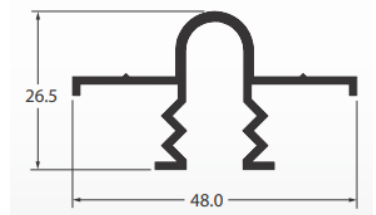
Perfil E – 364
