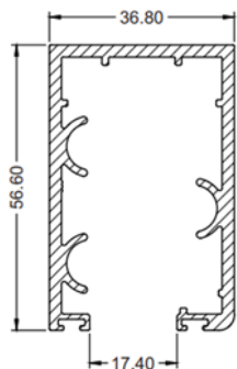
SP- 0298 Trilho triplo sup
