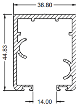
SP – 0297 Trilho duplo inf
