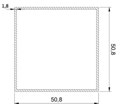
Tubo 2x2 PESADO
