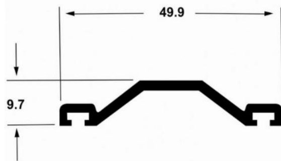
PERFIL TRAPÉZIO
