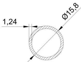
Tubo 5/8"
