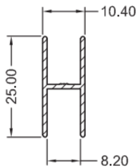
Perfil H – SP - 0118
