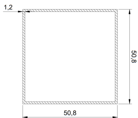
Tubo 2x2 INTERMEDIÁRIO
