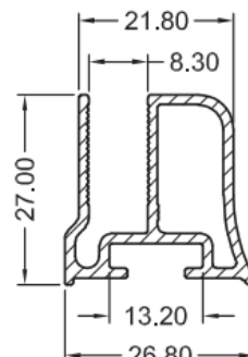
SP – 0595 Leito Olga de 8mm
