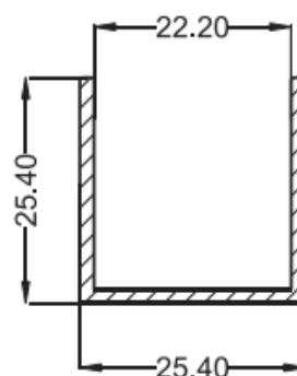
Perfil U 0829-A
