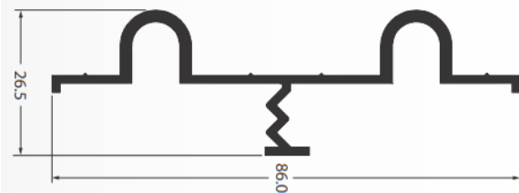
Perfil E – 365
