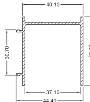
SP – 0295 Perfil U de regulagem
