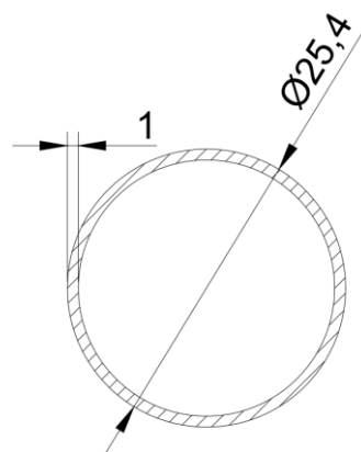
Tubo 1"
