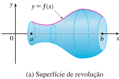
(a) Superfície de revolução
