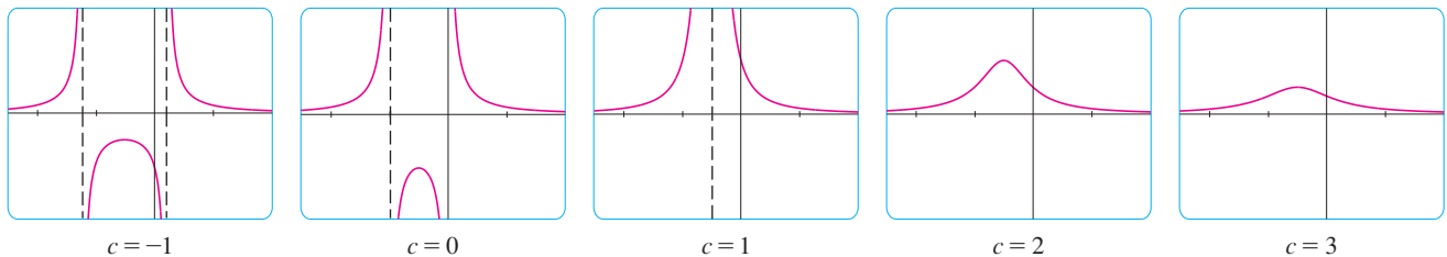
FIGURA 21 A família das funções f(x) = 1/(x^2 + 2x + c)
