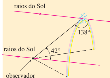
Formação do arco-íris principal
