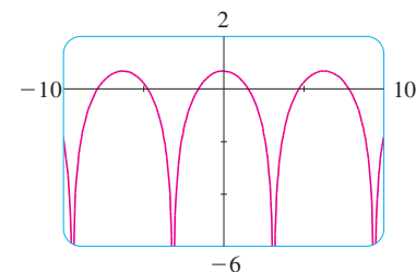
FIGURA 7 y = \ln(1 + \cos x)
