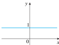
(b) y = 1^x
