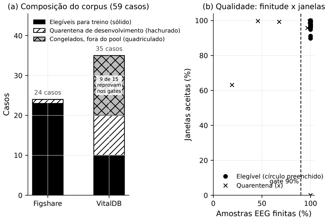
Figura 7. Composição e qualidade do corpus.
