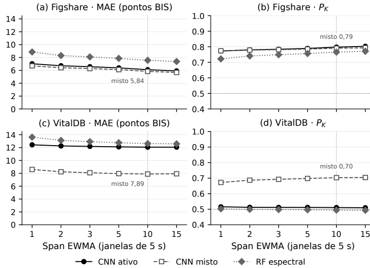
Figura 8. Varredura de spans do EWMA causal por braço: MAE e P_K no Figshare e no VitalDB.
