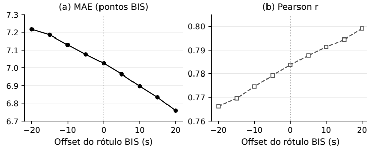
Figura 7. Sensibilidade ao offset do rótulo; eixos ampliados (variação total \leq 0,5 ponto de MAE e 0,04 de Pearson).
