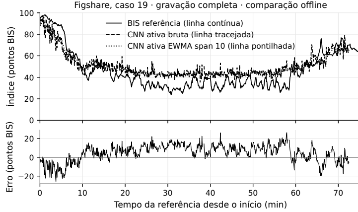
Figura 3. Trajetória offline do caso 19: referência e predição bruta (topo) e erro por janela (base).
