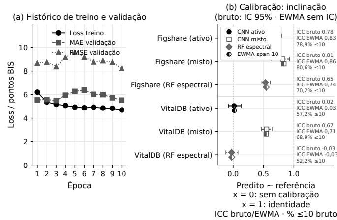
Figura 10. Treinamento do ativo e calibração por braço.
