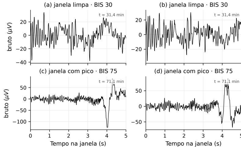
Figura 2. Janelas reais do caso 19 antes (bruto, em \mu V ) e depois do pipeline causal; a janela com pico mostra o efeito do clip, filtro e escala.
