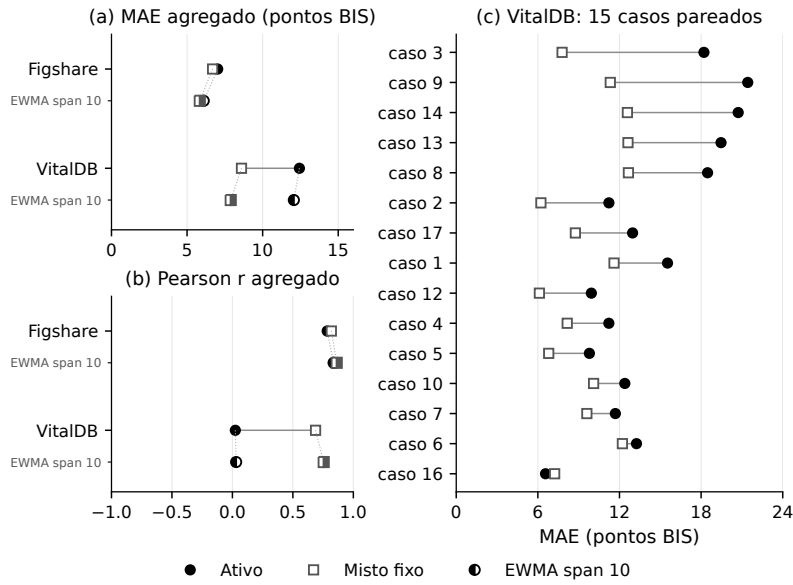
Figura 4. Agregados por janela e MAE pareado por caso; em (c), cada ponto é um caso e linhas à esquerda indicam menor MAE do misto.
