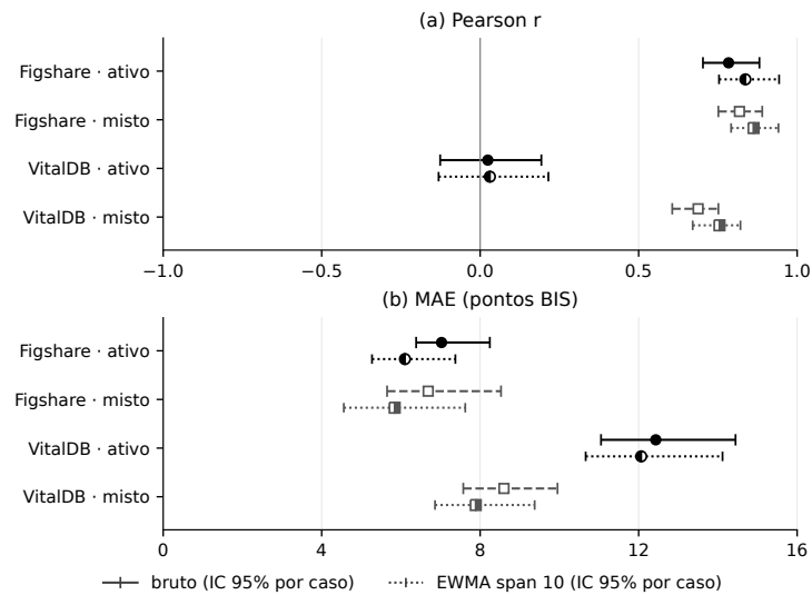
Figura 6. Bootstrap agrupado por caso.
