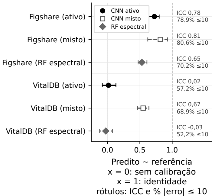
(b) Calibração: inclinação (IC 95% por caso)
