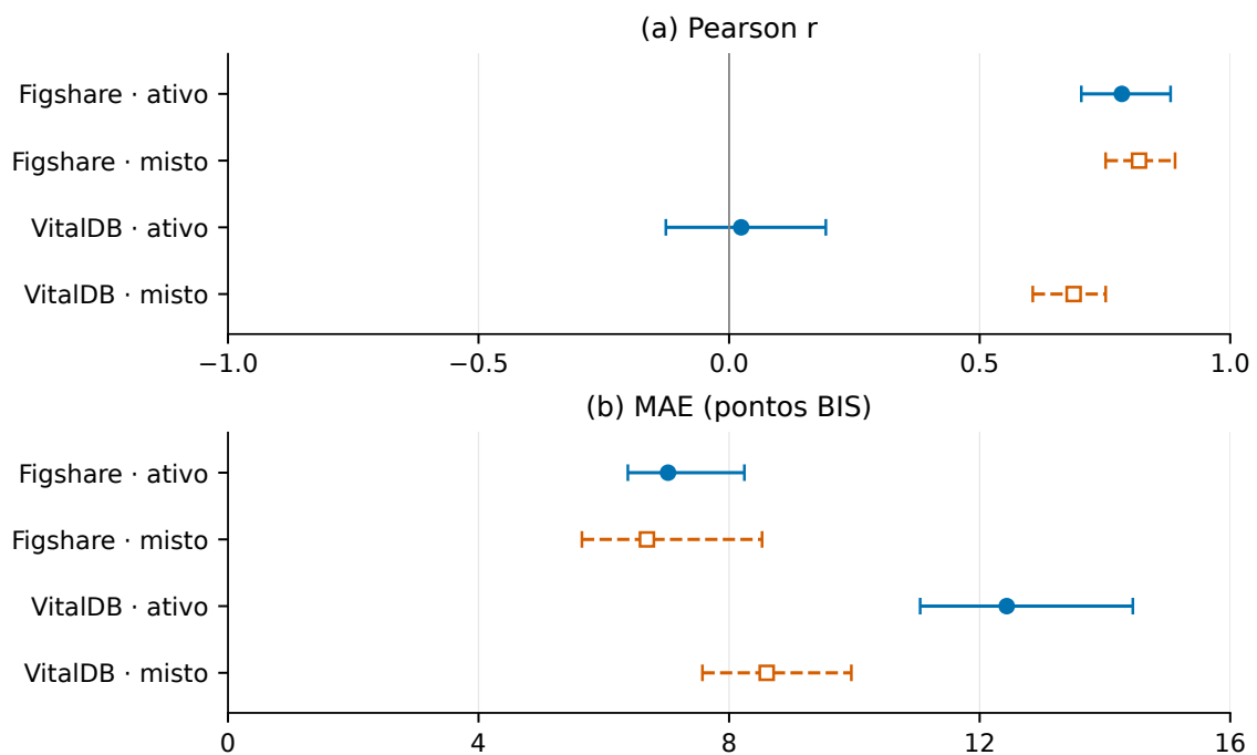
Figura 4. Métricas observadas (marcadores) e intervalos percentis de 95% (barras) do bootstrap por caso ( B = 1.000 , seed 42). Cada caso sorteado contribui com todas as janelas. O n = 5 do Figshare limita a leitura [Guimarães sd].
