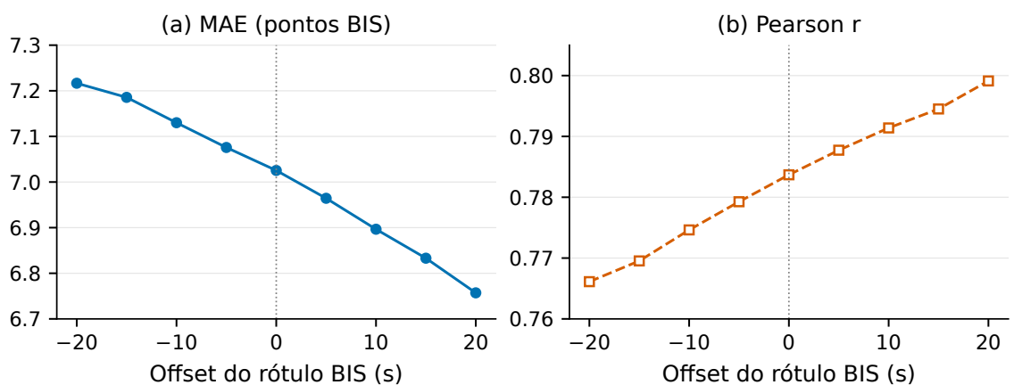
Figura 5. Sensibilidade pós-hoc ao alinhamento do rótulo em cinco casos Figshare. O número de janelas varia de 5.503 a 5.525, sem restrição a suporte comum. A linha vertical indica o padrão 0 s. A análise sem retreino gera hipótese e não seleciona atraso. Fonte: reports/offset_sensitivity.json [Guimarães sd].
