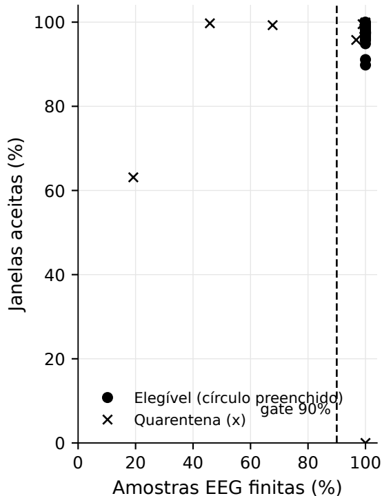
(b) Qualidade: finitude x janelas
