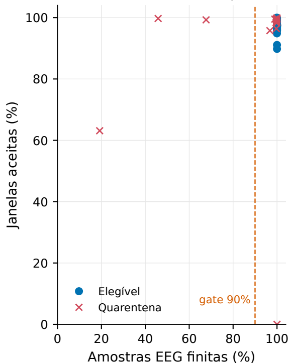
(b) Qualidade: finitude x janelas
