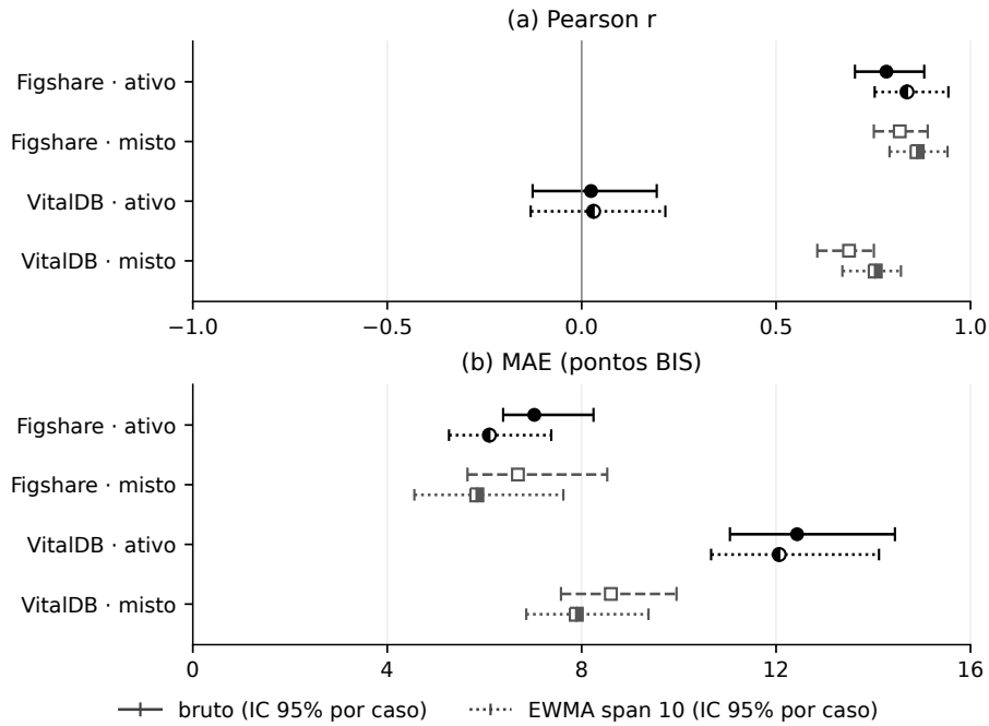
Figura 5. Bootstrap agrupado por caso.
