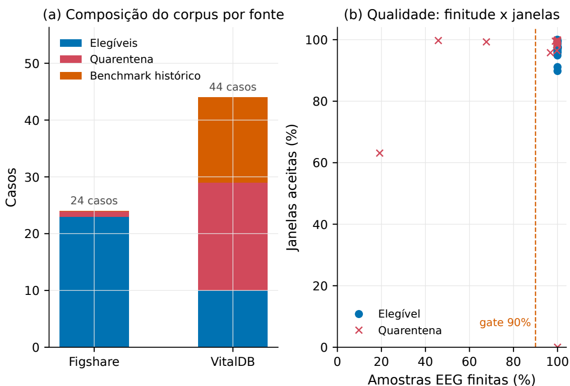
Figura 7. Composição e qualidade do corpus de desenvolvimento. (a) Casos por fonte, separando elegíveis, quarentena e benchmark histórico; a soma rotulada é o total de arquivos da fonte. (b) Fração de amostras de EEG finitas contra fração de janelas aceitas; a linha tracejada marca o gate de 90% de finitude. Gates e contagens vêm de reports/corpus/_manifest.json [Guimarães sd].
