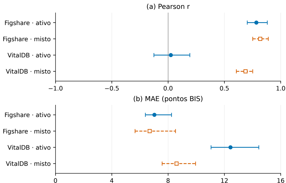
Figura 5. Métricas observadas (marcadores) e intervalos percentis de 95% (barras) do bootstrap por caso ( B = 1.000 , seed 42). Cada caso sorteado contribui com todas as janelas. O n = 5 do Figshare limita a leitura [Guimarães sd].
