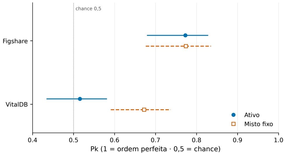
Figura 4. Probabilidade de predição P_K (Figshare 5/5.523; VitalDB 15/38.730), ativo vs misto, com IC 95% por reamostragem de casos ( B = 1.000 , seed 42). A linha pontilhada marca o acaso em 0,5. O indicador é a estimativa da CNN e a escala observada é o BIS de referência do monitor, não um desfecho de resposta ao estímulo [Smith et al. 1996, Guimarães sd].
