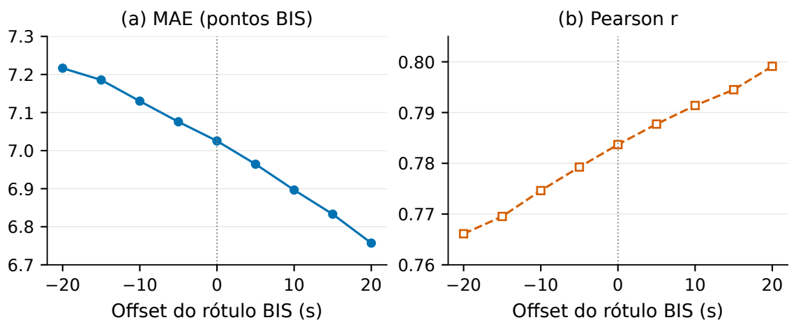
Figura 6. Sensibilidade pós-hoc ao alinhamento do rótulo em cinco casos Figshare. O número de janelas varia de 5.503 a 5.525, sem restrição a suporte comum. A linha vertical indica o padrão 0 s. A análise sem retreino gera hipótese e não seleciona atraso. Fonte: reports/offset_sensitivity.json [Guimarães sd].
