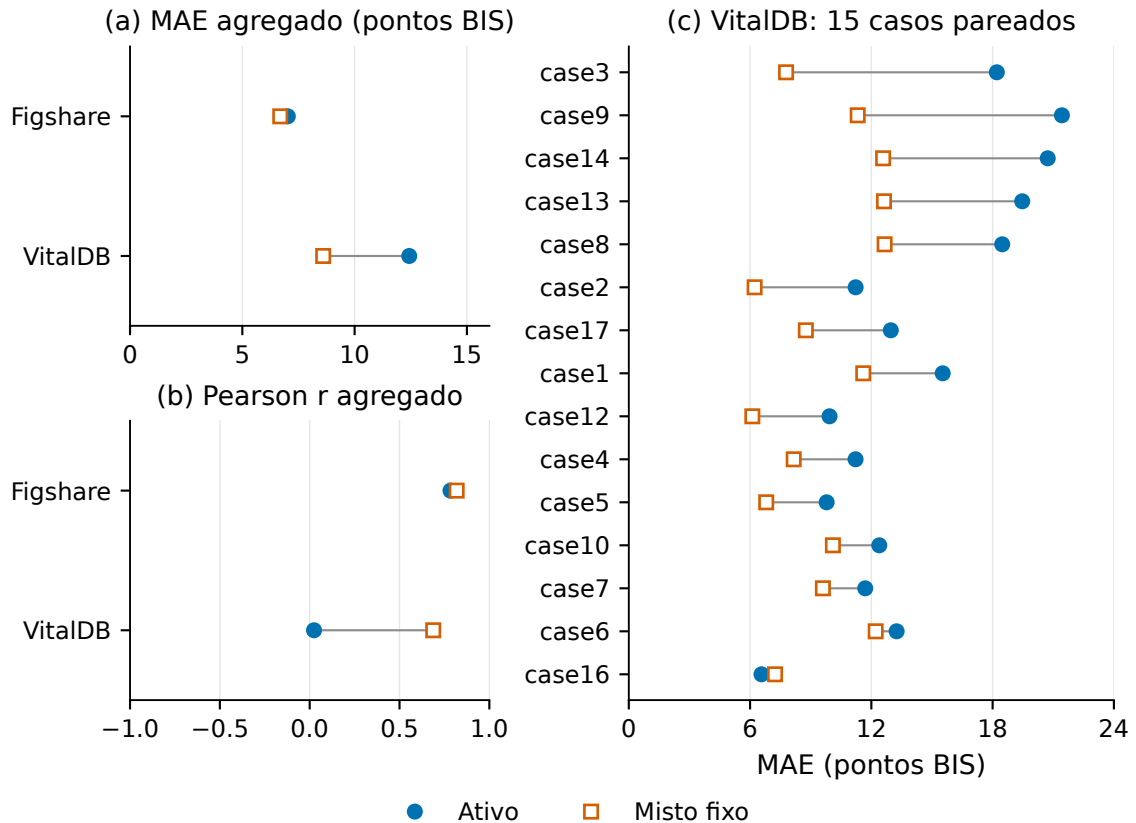
Figura 3. Agregados por janela no Figshare (5 casos/5.523 janelas) e VitalDB (15/38.730) e MAE pareado por caso, ordenado pela diferença misto menos ativo. O ativo viu só o Figshare; o misto já viu outros participantes VitalDB. Pontos e linhas vêm dos quatro relatórios citados no texto; 14/15 casos melhoram, mas o caso 16 piora cerca de 0,67 [Guimarães sd].
