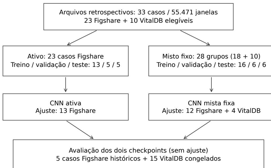
Figura 1. Fluxo retrospectivo auditável do BrainSniffer, a partir de arquivos existentes. A separação por grupo impede que janelas do mesmo grupo atravessassem partições; no Figshare, o grupo é o caso. O pool elegível de 33 casos não é o corpus fixo de 28 grupos, que exclui os cinco casos históricos e se divide em 16/6/6. As setas finais indicam avaliação, nunca treino. Fontes internas [Guimarães sd]; o benchmark VitalDB do misto não é confirmatório.
