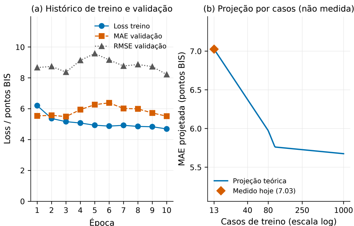
Figura 8. Apoio de treinamento e planejamento. (a) Histórico de treino e validação do checkpoint ativo por época: perda de treino (adimensional) e MAE/RMSE de validação (pontos BIS). (b) Projeção teórica de MAE por número de casos de treino, em escala logarítmica, ancorada no único valor medido (13 casos, MAE 7,03): cenário de planejamento, não curva medida [Guimarães sd].
