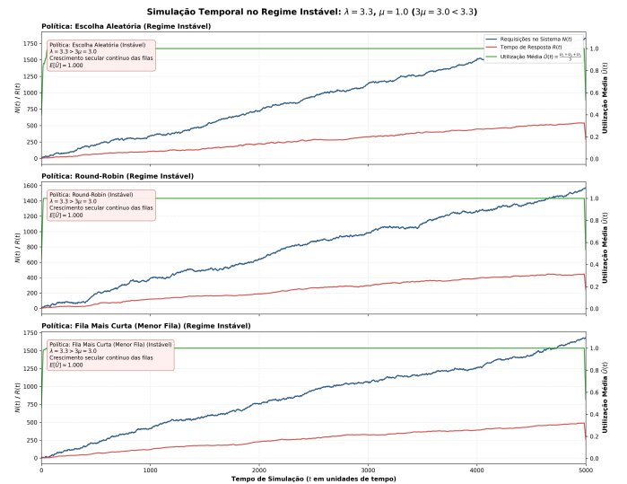
Fig. 4. Simulação temporal no regime instável ( \lambda = 3,3 , 3\mu = 3,0 ): crescimento ilimitado de N(t) e R(t) .
