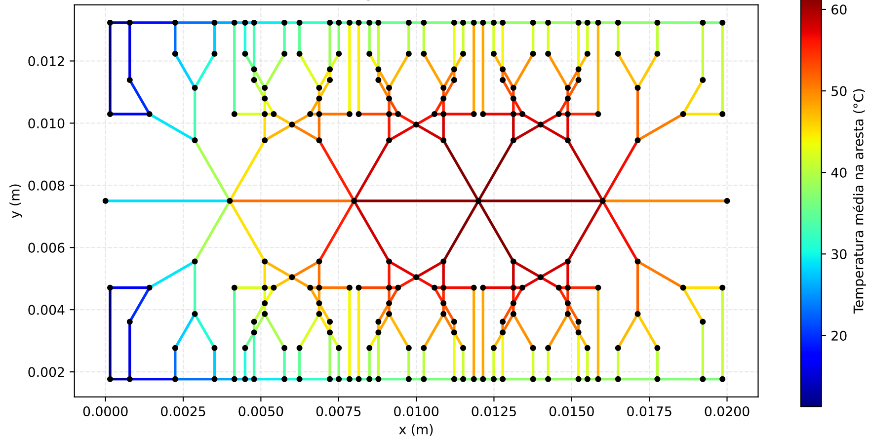
Distribuição térmica integrada nas arestas da rede (N = 1000)
