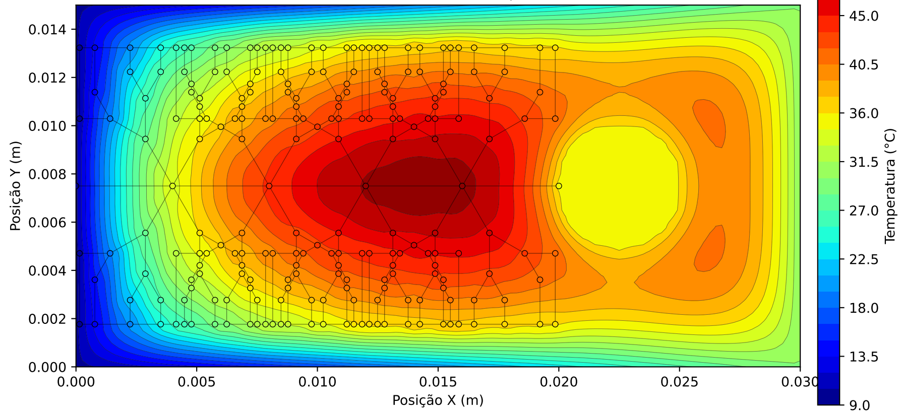
Campo Térmico 2D - Malha 121x61 | d_{max} = 0.00025 m
