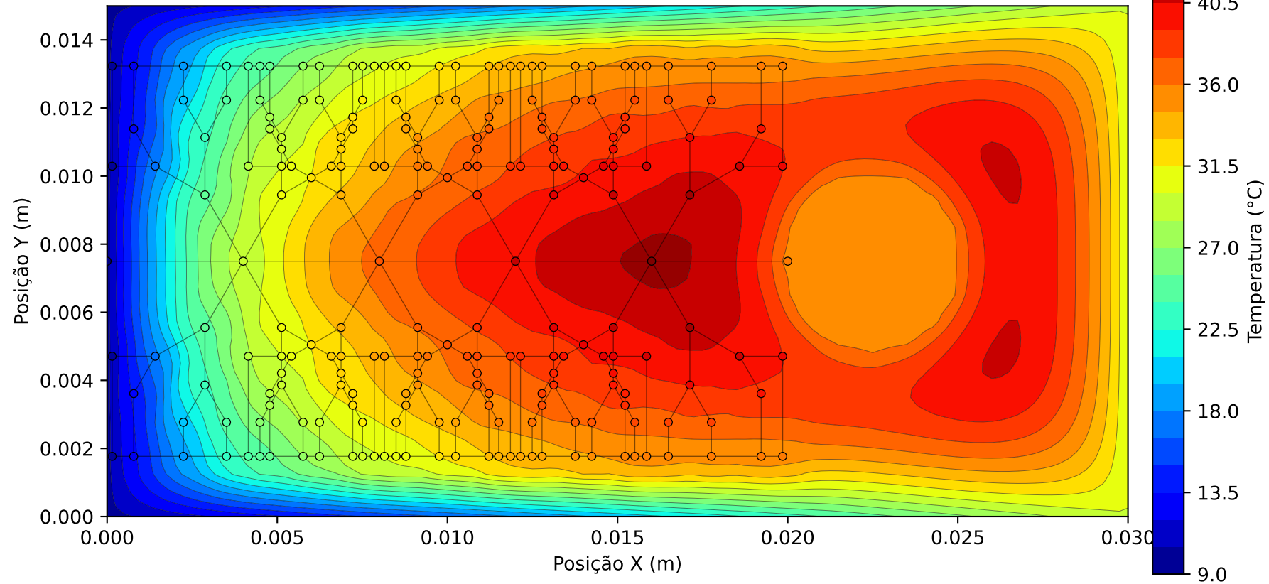
Campo Térmico 2D - Malha 121x61 | d_{max} = 0.0005 m
