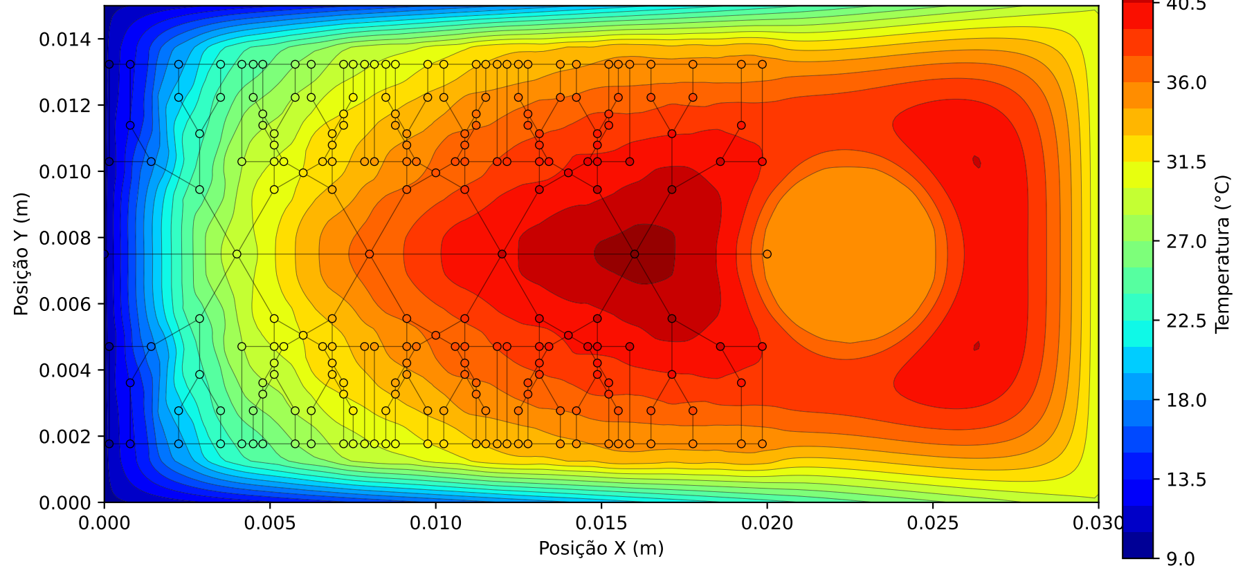
Campo Térmico 2D - Malha 241x121 | d_{max} = 0.0005 m
